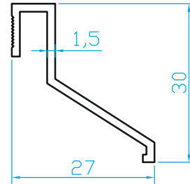
K558 GEÇME DAMLALIK (0.225 Kg/m)
