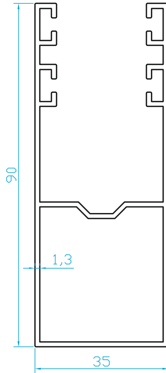
K6714 90mm PANJUR YAN "U" (1.060 Kg/m)
