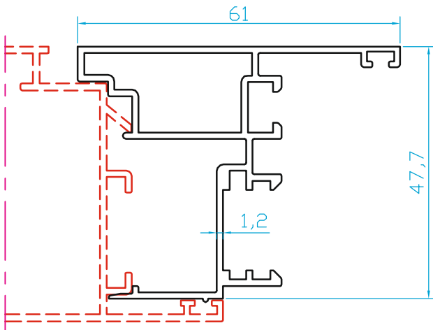
K7893 YALITIMSIZ OVAL SERİ ÇİFT KAPI ADAPTÖRÜ (0.770 Kg/m)
