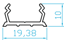
K522 20'LİK GRİYAJ TABANI (0.130 Kg/m)
