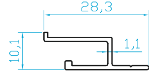
K603 ASMA TAVAN 0.151 Kg/m
