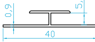
K6872 ÖZEL BİRLEŞİM (0.150 Kg/m)
