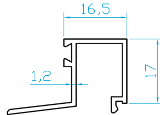
K520 ALDOKS ISICAM ÇİTA (0.205 Kg/m)
