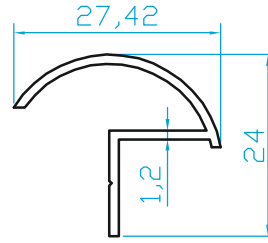
K4562 0.195 Kg/m
