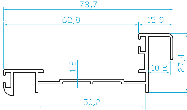
K6806 ÇELİK KAPI PROFİLİ (0.540 Kg/m)
