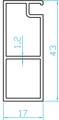
K633 KAPI SİNEKLİK (0.442 Kg/m)
