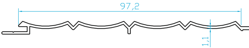
K745 DESENLİ YAPRAK LAMBRI (0.400 Kg/m)
