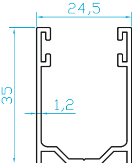
K6719 FİTİLLİ PANJUR "U" (0.370 Kg/m)
