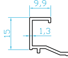
K6834 GİZLİ FİTİL SİNEKLİK ÇİTA (0.160 Kg/m)
