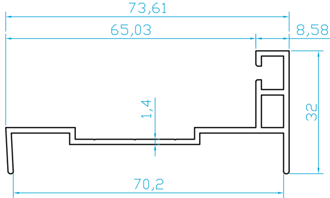
K4633 ÇELİK KAPI PROFİLİ (0.570 Kg/m)
