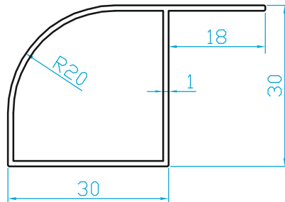
K6727 30x30 OVAL KÖŞE (0.345 Kg/m)
