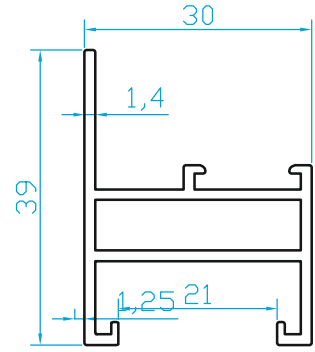
K6735 KANAT (0.495 Kg/m)
