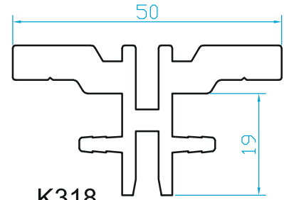
K318 MAĞAZA DEKORASYON (1.300 Kg/m)
