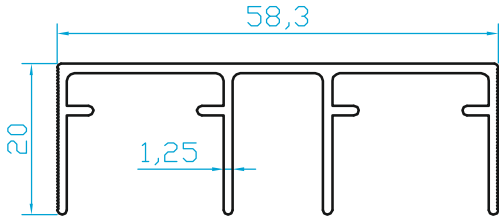
K6709 SÜRME KAPAK ÜST RAY (0.490 Kg/m)
