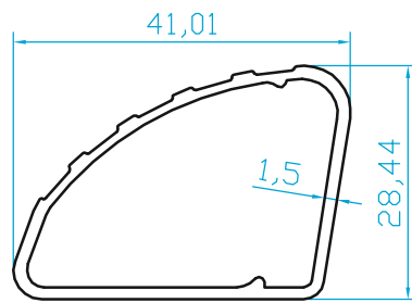
K6849 OTO PORBAGAJ PROFİLİ (0.450 Kg/m)
