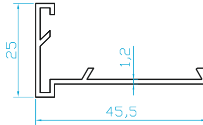
K652 ALDOKS TIRNAK (0.275 Kg/m)
