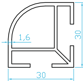
K599 PORTATİF KÖŞE DÖNÜŞ (0.550 Kg/m)
