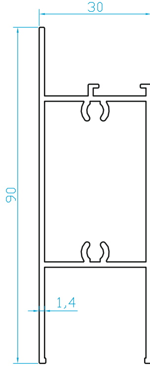
K6734 FOTOSSEL KAPI KANAT (0.945 Kg/m)
