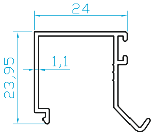
K449 ÇITA (0.260 Kg/m)
