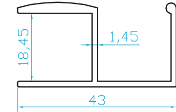
K6626 MOBİ DEKO KULP PRF. (0.475 Kg/m)
