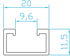
K5525 DİLARA VİTRİN (0.180 Kg/m)
