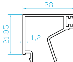
K7897 YALITIMSIZ OVAL SERİ TEKCAM ÇİTASI (0.315 Kg/m)
