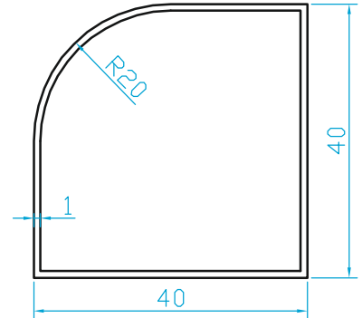
K693 40x40 OVAL KÖŞE (0.400 Kg/m)
