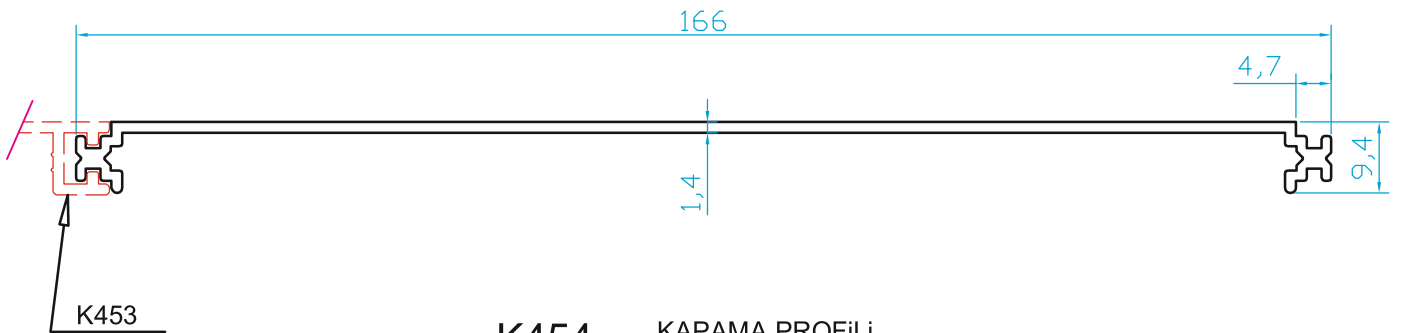
K454 KAPAMA PROFİLİ (0.750 Kg/m) (ORJ. NO:)14-3093
