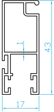
K607 SÜRME SİNEKLİK (0.410 Kg/m)
