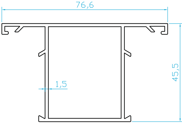
K502A GENİŞ ALDOKS DÜZ KAYIT (0.925 Kg/m)
