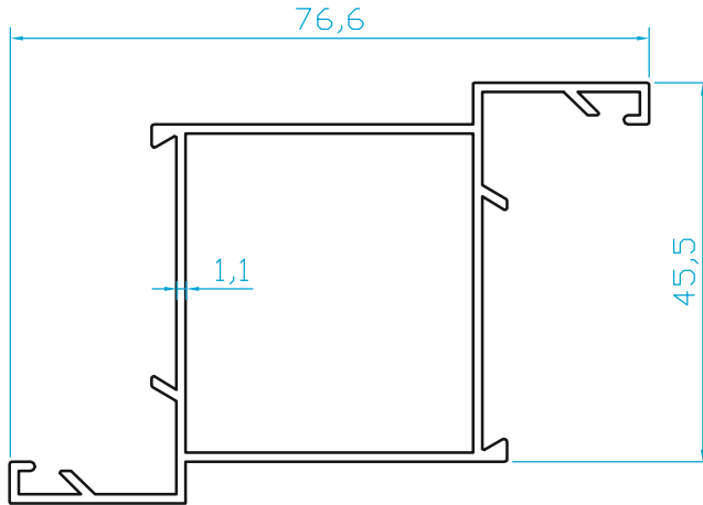
K509 GENİŞ ALDOKS FUGALI KANAT (0.710 Kg/m)
