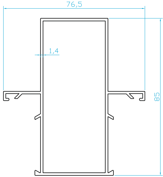
K596 ALDOKS FUGALI BÜYÜK KAYIT (1.090 Kg/m)
