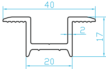
K4601 ORTA TUTUCU PROFİL 0.390 Kg/m
