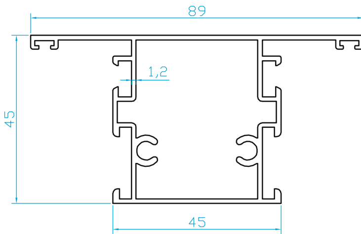
K7890 YALITIMSIZ OVAL SERİ GENİŞ ORTA KAYIT PROFİLİ (1.050 Kg/m)
