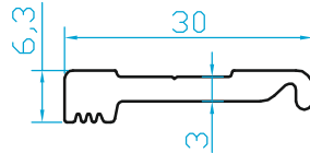
K4606 AŞIK PROFİLİ SABİTLEME TIRNAĞI 0.310 Kg/m
