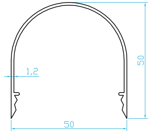
K523 50'LİK GRİYAJ ÇİTASI (0.450 Kg/m)
