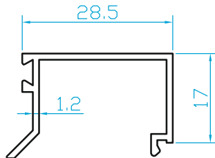
K519 ALDOKS TEKCAM ÇİTA (0.220 Kg/m)
