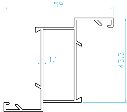
K512 DAR ALDOKS FUGALI KANAT (0.600 Kg/m)
