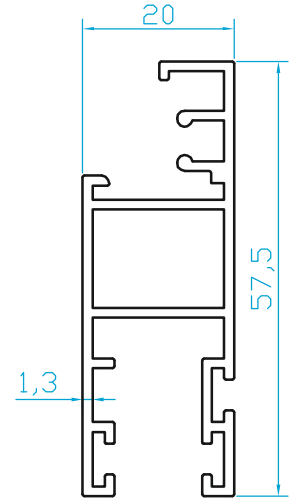
K6833 GİZLİ FİTİL SİNEKLİK KANAT (0.665 Kg/m)
