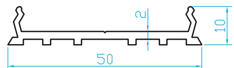
K524 50'LİK GRİYAJ GEÇMESİ (0.360 Kg/m)
