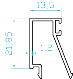
K7895 YALITIMSIZ OVAL SERİ ISICAM ÇİTASI (0.240 Kg/m)
