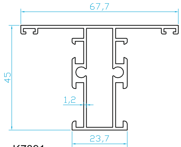
K7891 YALITIMSIZ OVAL SERİ DAR ORTA KAYIT PROFİLİ (0.860 Kg/m)
