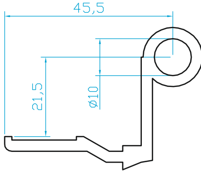
K751 MENTEŞE (KANAT) (0.885 Kg/m)
