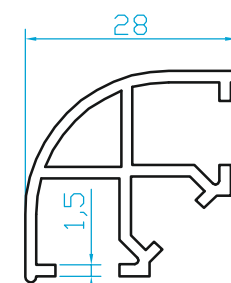
K676 3D KÖŞE DÖNÜŞ (0.290 Kg/m)
