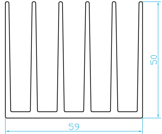
K6828 SOĞUTUCU PROFİLİ (2.090 Kg/m)
