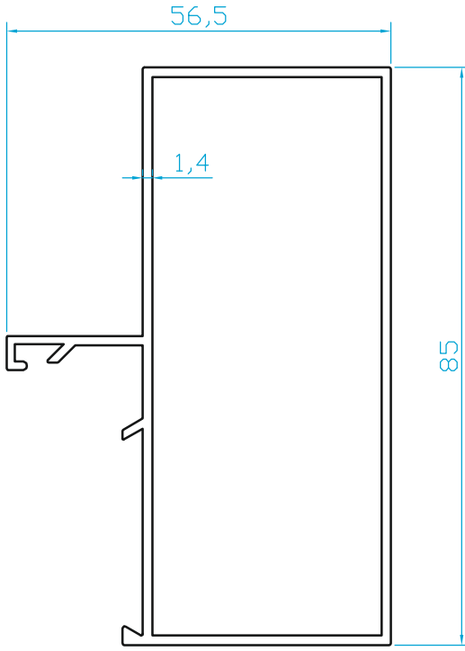
K595 ALDOKS FUGALI BÜYÜK KASA (1.050 Kg/m)
