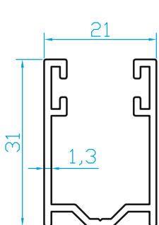
K6720 FİTİLLİ PANJUR "U" (0.362 Kg/m)
