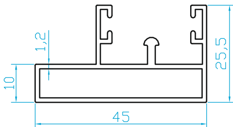
K6657 SÜRME SİNEKLİK KASA (0.540 Kg/m)
