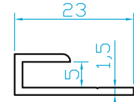
K154 BİTİM PROFİLİ (0.160 Kg/m)
