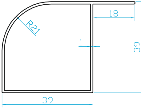
K6725 39x39 OVAL KÖŞE (0.445 Kg/m)
