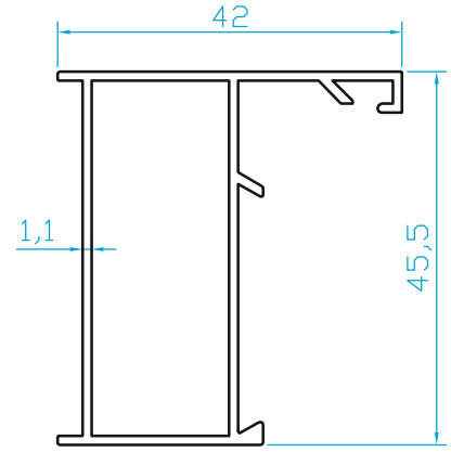
K504 DAR ALDOKS DÜZ KASA (0.500 Kg/m)
