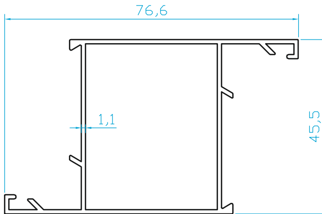
K503 GENİŞ ALDOKS DÜZ KANAT (0.700 Kg/m)
