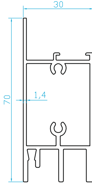
K327 FOTOSSEL KAPI ETEK (1.050 Kg/m)
