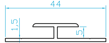
K153 ÖZEL BİRLEŞİM (0.275 Kg/m)
