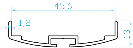
K574 ÇARPMA KAPI DIŞ KASA (0.260 Kg/m)
