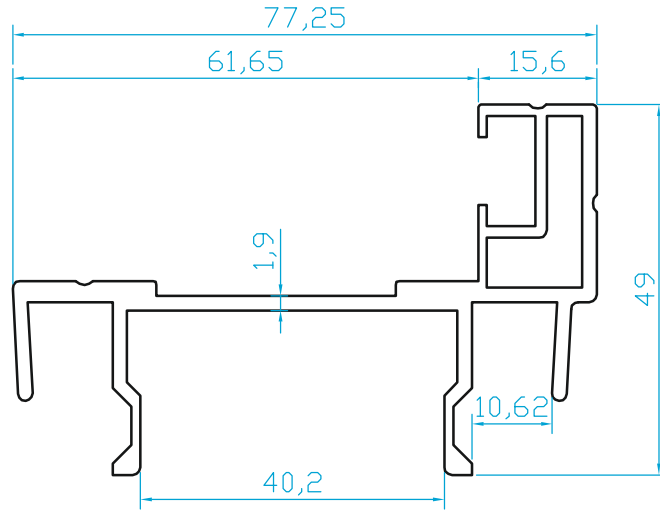
K4510 ÇELİK KAPI PROFİLİ (1.200 Kg/m)
