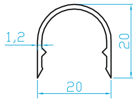
K521 20'LİK GRİYAJ (0.165 Kg/m)
