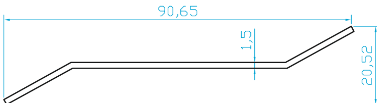
K267 ÖZEL YAPRAK MENFEZ (0.410 Kg/m)
