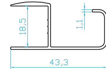
K1590 MOBİ DEKO KULP PRF. (0.335 Kg/m)
