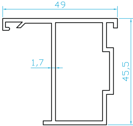
K859 DÜZ ALDOKS PİVOT ADAPTÖR (0.810 Kg/m)
