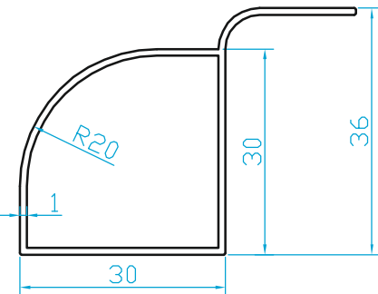
K6764 30x30 OVAL KÖŞE (0.355 Kg/m)
