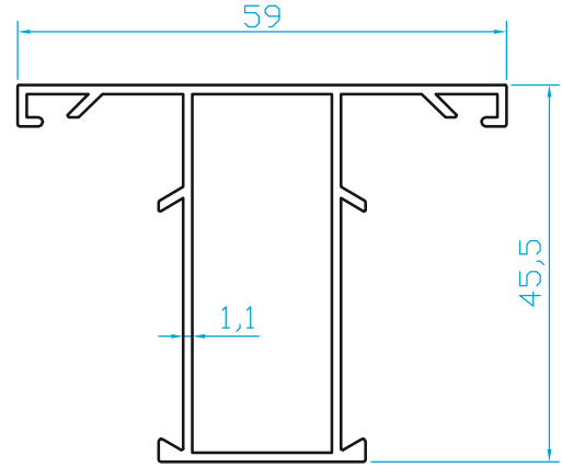
K505 DAR ALDOKS DÜZ KAYIT (0.600 Kg/m)
