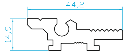
K1543 0.790 Kg/m
