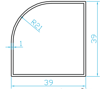
K6726 39x39 OVAL KÖŞE (0.395 Kg/m)
