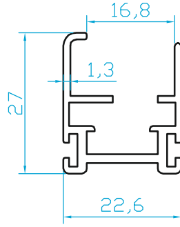
K1541 SÜRME KANAT 0.385 Kg/m
