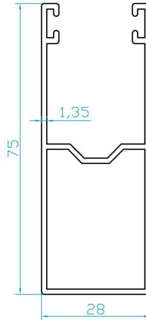
K6715 PANJUR YAN "U" (0.820 Kg/m)
