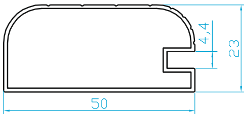
K6708 CAM KÖŞE PROFİLİ (0.410 Kg/m)
