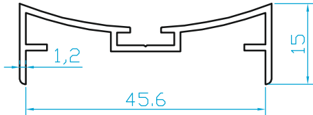
K573 ÇARPMA KAPI İÇ KASA (0.305 Kg/m)
