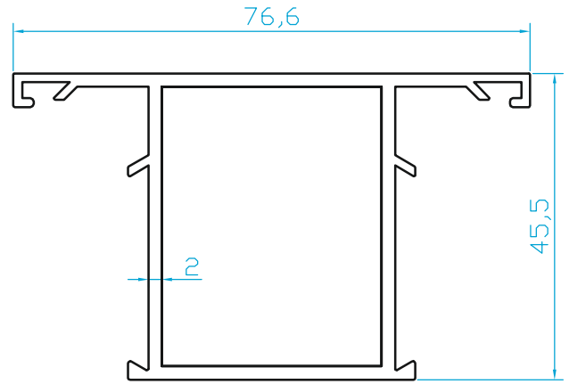
K502B GENİŞ ALDOKS DÜZ KAYIT (1.170 Kg/m)
