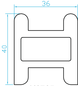
K6765 ASANSÖR PROFİLİ (1.795 Kg/m)
