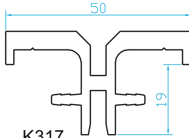
K317 MAĞAZA DEKORASYON (1.120 Kg/m)
