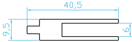
K319 ÖZEL PROFİL 0.550 Kg/m
