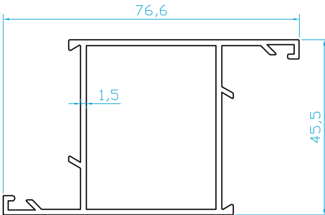
K503A GENİŞ ALDOKS DÜZ KANAT (0.925 Kg/m)
