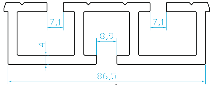
K6768 ASANSÖR PROFİLİ (2.460 Kg/m)
