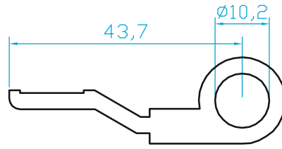
K752 MENTEŞE (KASA) (0.765 Kg/m)
