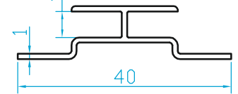
K6873 ÖZEL BİRLEŞİM (0.185 Kg/m)
