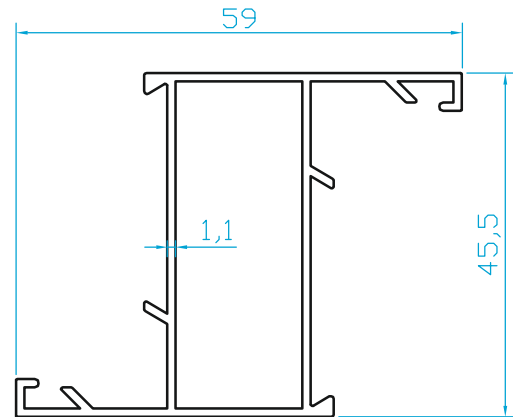
K506 DAR ALDOKS DÜZ KANAT (0.600 Kg/m)
