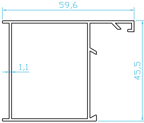
K501 GENİŞ ALDOKS DÜZ KASA (0.600 Kg/m)
