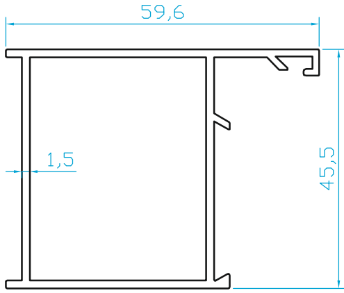
K501A GENİŞ ALDOKS DÜZ KASA (0.810 Kg/m)
