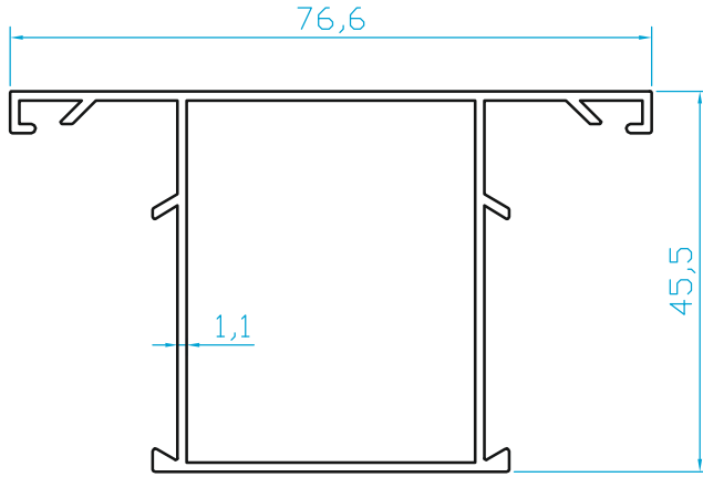
K502 GENİŞ ALDOKS DÜZ KAYIT (0.700 Kg/m)
