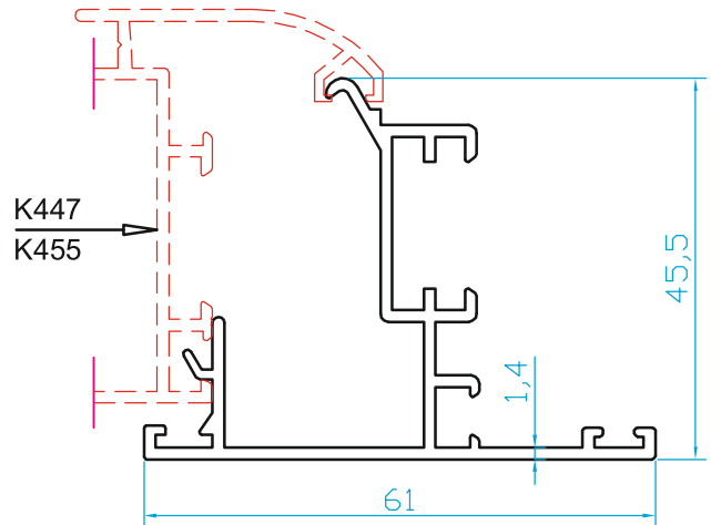
K448 ADAPTÖR (0.670 Kg/m)
