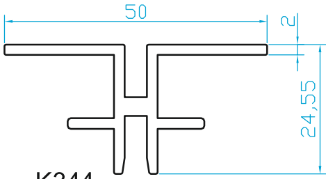
K344 MAĞAZA DEKORASYON (0.700 Kg/m)
