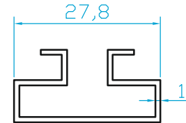
K873 MOBİLYA DEKO. (0.215 Kg/m)
