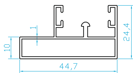
K6657 A SÜRME SİNEKLİK KASA (0.460 Kg/m)
