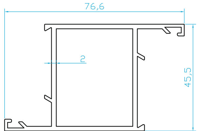
K503B GENİŞ ALDOKS DÜZ KANAT (1.170 Kg/m)
