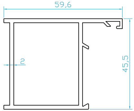
K501B GENİŞ ALDOKS DÜZ KASA (1.050 Kg/m)
