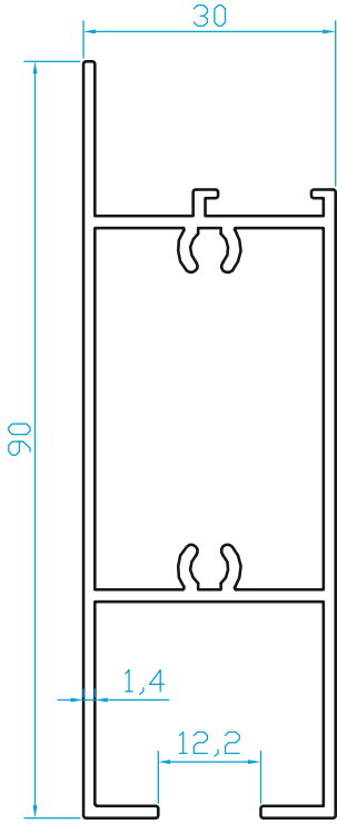
K6733 FOTOSSEL KAPI KANAT (0.998 Kg/m)
