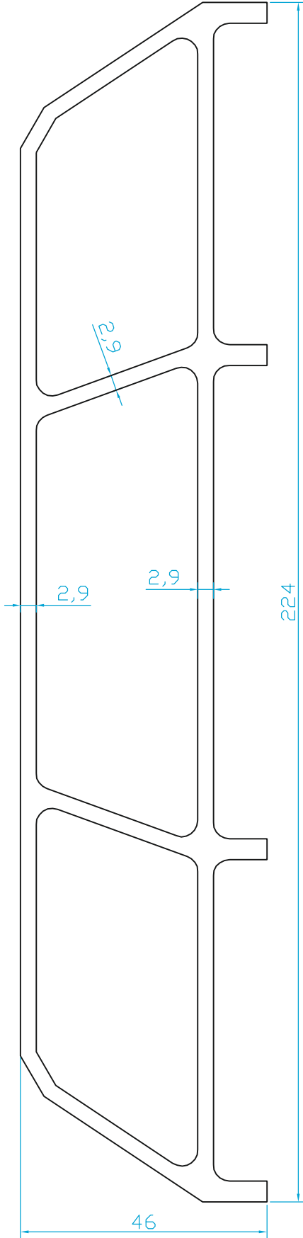
K1545 PALET PROFİLİ (2.820 Kg/m)
