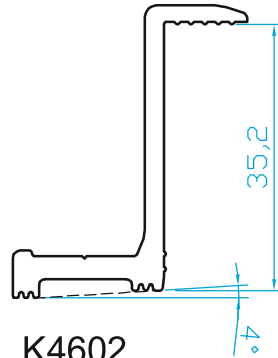
K4602 KENAR TUTUCU PROFİL 0.495 Kg/m
