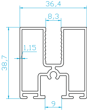
K1970 KARE TEKCAM BAZA 0.815 Kg/m
