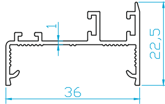
K4619 SIZDIRMAZLIK PRF. (0.300 Kg/m)
