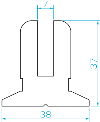
K2316 KÜPEŞTE AKSESUAR 1.900 Kg/m
