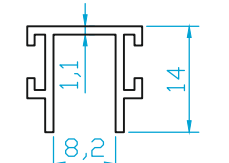
K4497 CAM TUTUCU 8 mm 0.157 Kg/m
