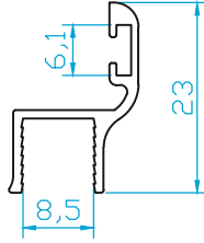
K4491 8mm CAM FİTİL 0.165 Kg/m
