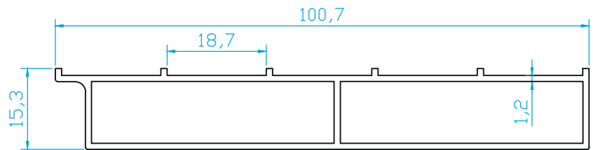
K4560 SÜRME FİX YAN KASA 0.770 Kg/m
