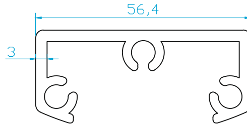
K266 KÜPEŞTE BAĞLANTI PROFİLİ 1.085 Kg/m
