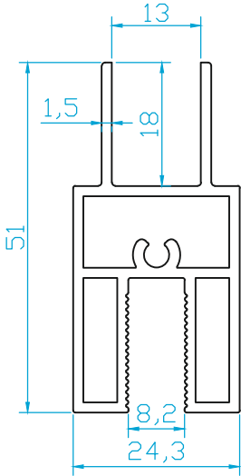
K4984 TEKCAM TUTUCU ZİNCİR ASKILI (0.830 Kg/m)
