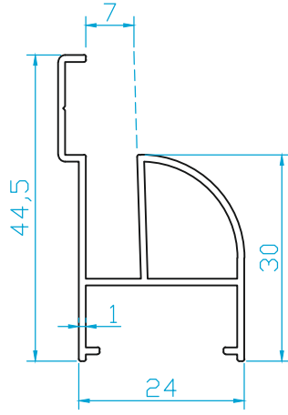
K2319 EKO TABAN PROFİLİ 0.365 Kg/m
