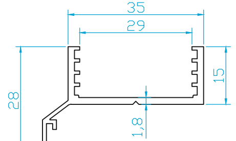
K4640 KANAT KARŞILIK (0.390 Kg/m)
