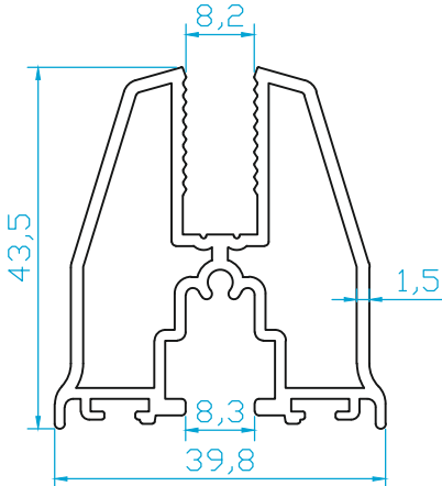
K4611 KATLANIR KANAT 0.935 Kg/m
