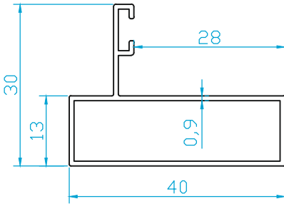
K4852 DiKME (0.325 Kg/m)
