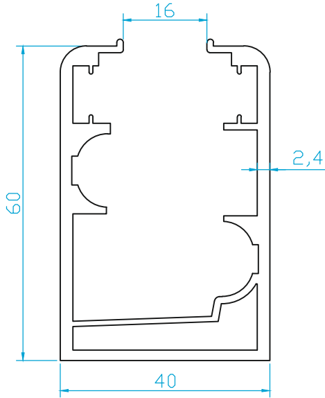
K4517 ÖZEL KASA (1.395 Kg/m)
