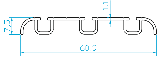
K4462 EŞİKSİZ ALT KASA (3LÜ) 0.340 Kg/m
