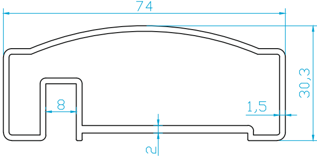
K2257 KÜPEŞTE BALKON PROFİLİ (0.960 Kg/m)
