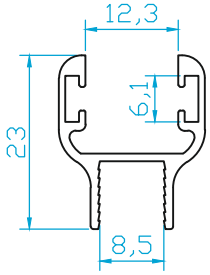
K4490 8mm CAM FİTİL 0.240 Kg/m
