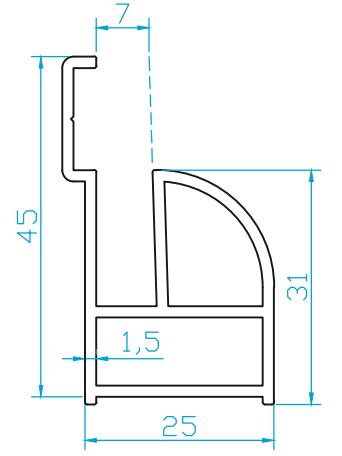
K2259 TABAN PROFİLİ 0.615 Kg/m
