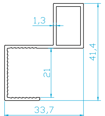
K1274 SPANYOLET KANAT 0.405 Kg/m
