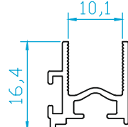
K4531 ÜST FİTİL 0.175 Kg/m
