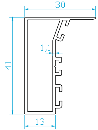
K1981 DİKME (MIKNATIS KANALLI) 0.445 Kg/m
