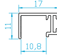
K2314 FİTİL PROFİLİ 0.120 Kg/m
