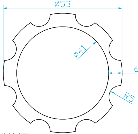
K287 Ø40 DEKO DİKME TABANI 1.850 Kg/m
