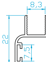
K4773 CAM FİTİL 0.140 Kg/m
