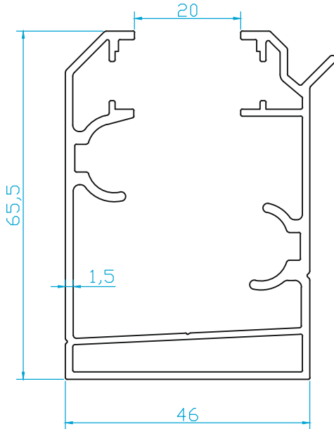
K4273 KASA PROFİLİ (DAMLALIKLI) 1.275 Kg/m
