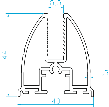
K4482 KANAT (0.900 Kg/m)
