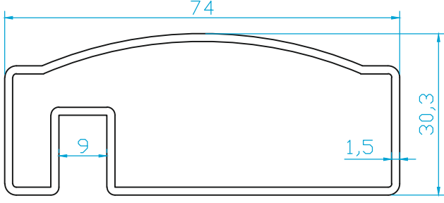
K2390 KÜPEŞTE BALKON PROFİLİ (0.960 Kg/m)
