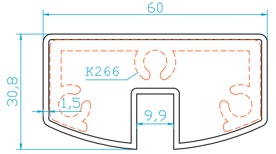
K2276 KÜPEŞTE BALKON PROFİLİ 0.800 Kg/m
