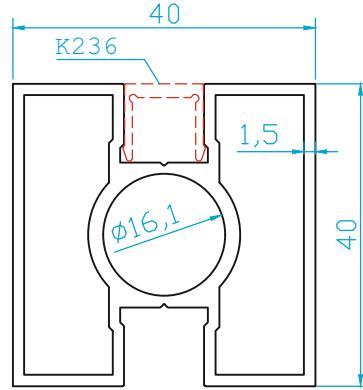
K235 KÜPEŞTE DİKME (1.040 Kg/m)
