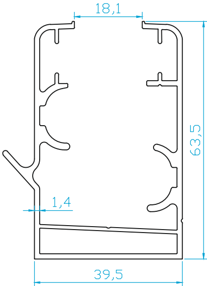
K4262 CAMBALKON KASA 1.110 Kg/m
