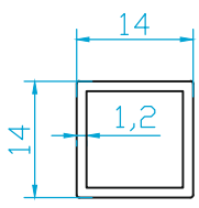
(K2323) 14X14 (0.175 Kg/m)
