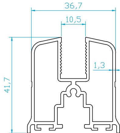
K4558 CAM BALKON KATLANIR KANAT (0.850 Kg/m)
