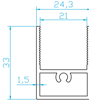
K4877 ÇİFTCAM TUTUCU (0.495 Kg/m)
