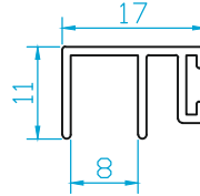
K2313 FİTİL PROFİLİ 0.140 Kg/m
