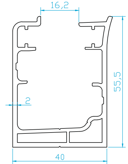
K1482 CAMBALKON KASA 1.165 Kg/m
