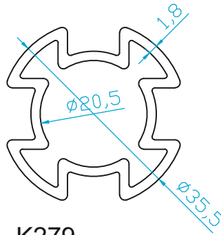
K279 DEKORATİF DiKME 0.760 Kg/m
