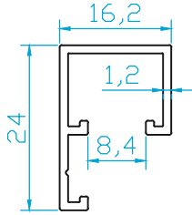
K4271 CAM KENAR 0.205 Kg/m
