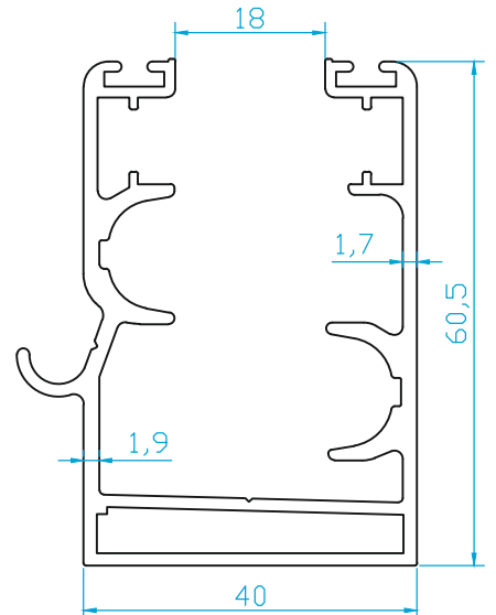
K4464 A DAMLALIKLI KASA HAFİF (1.350 Kg/m)
