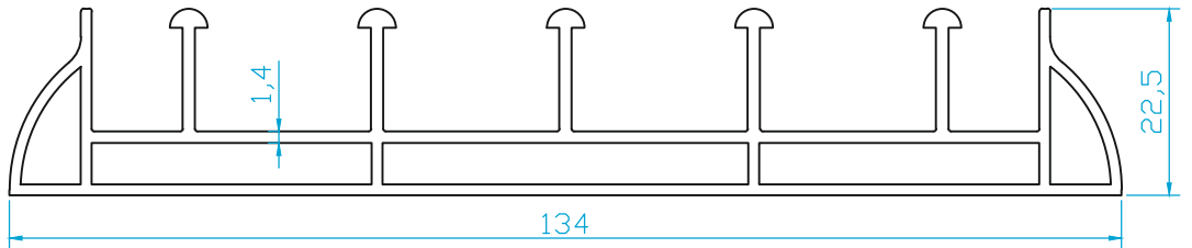
K4573 CAM BALKON SÜRME KIZAK 20 mm (1.590 Kg/m)
