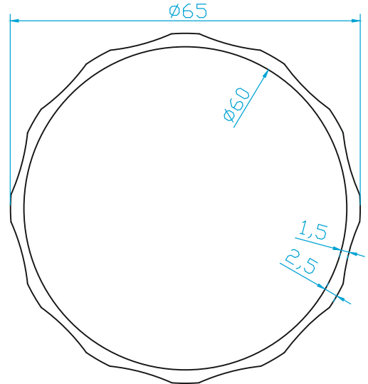
K227 Ø65 KÜPEŞTE DEKORATİF BORU 1.300 Kg/m
