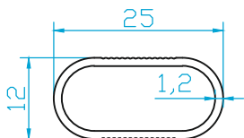
K238 A DEKOR 0.195 Kg/m
