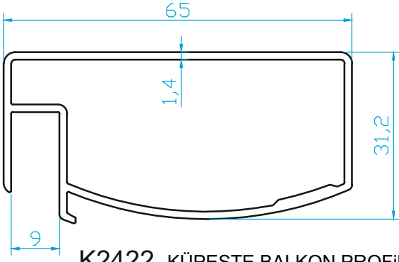
K2422 KÜPEŞTE BALKON PROFİLİ (0.785 Kg/m)
