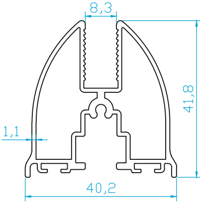
K4263 CAMBALKON KANAT 0.750 Kg/m
