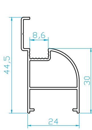
K2448 EKO TABAN PROFİLİ 0.345 Kg/m
