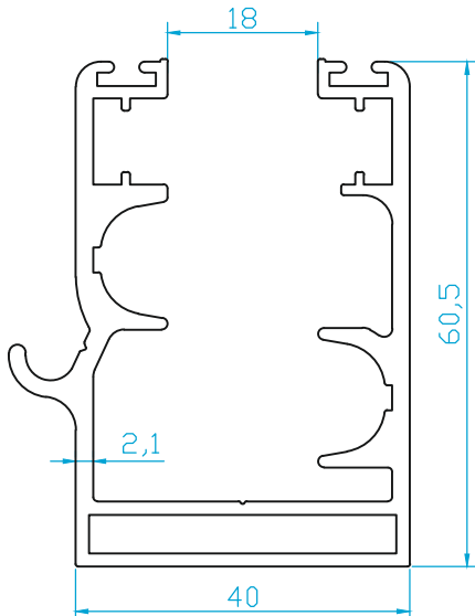
K4464 DAMLALIKLI KASA (1.510 Kg/m)
