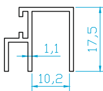
K4495 CAM TUTUCU 10mm 0.200 Kg/m
