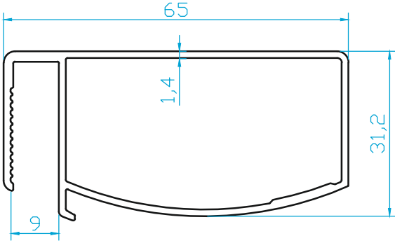
K2446 KÜPEŞTE BALKON PROFİLİ (0.755 Kg/m)
