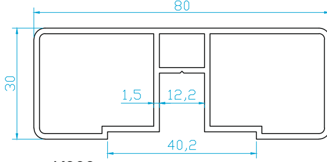
K393 KÜPEŞTE KORKULUK (1.070 Kg/m)
