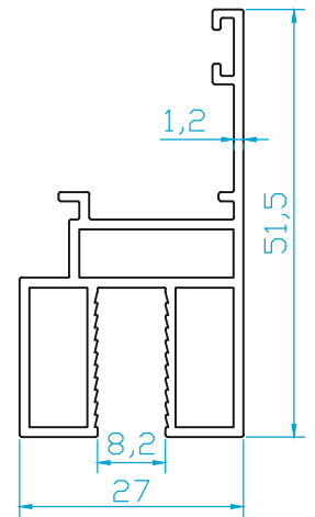
K1894 SPANYOLET KANAT KARŞILIK 0.615 Kg/m
