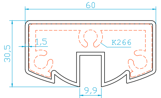
K265 KÜPEŞTE BALKON PROFİLİ 0.820 Kg/m
