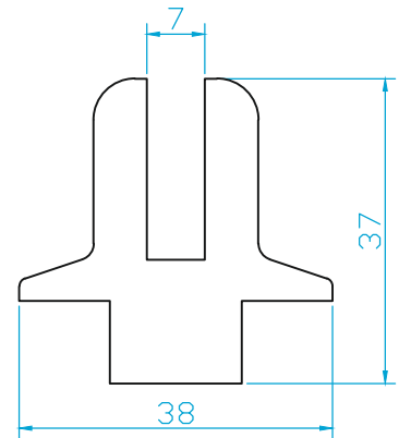
K2362 KÜPEŞTE AKSESUAR 1.660 Kg/m
