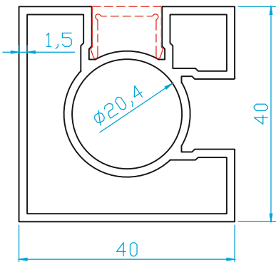
K253 KÖŞE DİKME (0.960 Kg/m)
