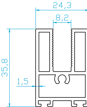
K1547 TEKCAM TUTUCU (0.735 Kg/m)
