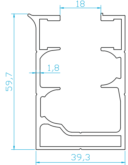
K1663 CAMBALKON KASA 1.230 Kg/m
