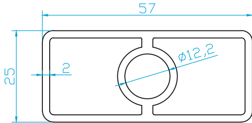
K2301 60x28 DEKO KUTU BAĞLANTI (K2300) (1.130 Kg/m)
