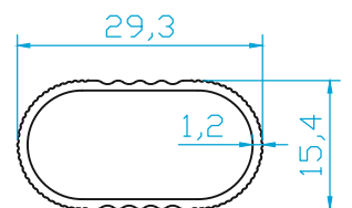
K1009 OVAL DEKO BORU 0.215 Kg/m
