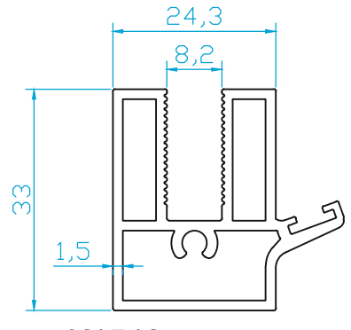
K1548 FİTİLLİ TEKCAM TUTUCU (0.755 Kg/m)
