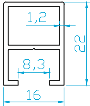
K2380 CAM KENAR 0.250 Kg/m
