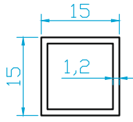
(K2427) 15X15 (0.190 Kg/m)
