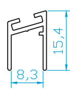
K2293 CAM TUTUCU 0.110 Kg/m
