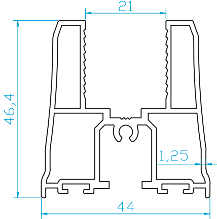
K4861 ISICAMLI KANAT 0.980 Kg/m
