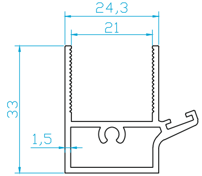
K4878 FİTİLLİ ÇİFTCAM TUTUCU (0.565 Kg/m)
