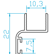
K4872 CAM FİTİL 10 mm 0.105 Kg/m
