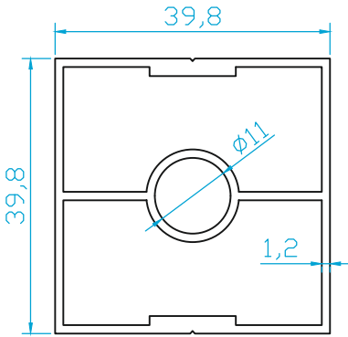
K274 KÜPEŞTE DİKME 0.810 Kg/m
