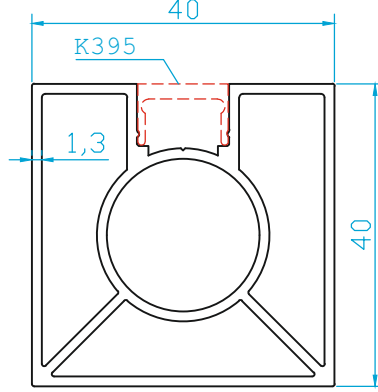
K394 KÜPEŞTE DİKME (0.935 Kg/m)
