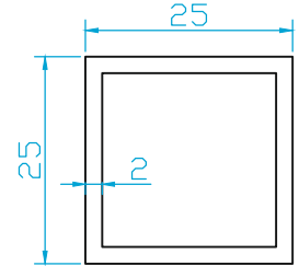
(K5547) 25X25 (0.500 Kg/m)
