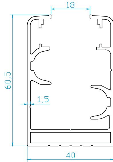
K1233 KASA PRF.(FIRTINA) 1.145 Kg/m
