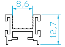
K4496 CAM KARŞILIK 8 mm 0.165 Kg/m
