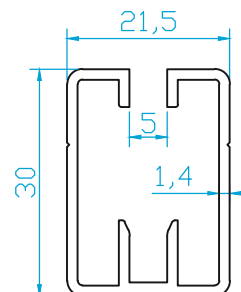
K2345 30x21.5 DEKO ÇEÇEVE (0.445 Kg/m)
