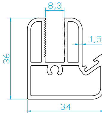
K1580 FİTİLLİ TEKCAM TUTUCU KISA MODEL 0.830 Kg/m
