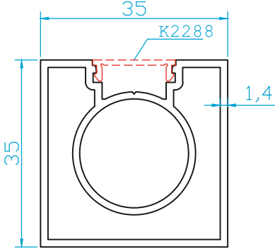
K2289 35x35 KÜPEŞTE DİKME 0.760 Kg/m
