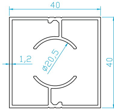
K2352 40x40 DİKME 0.725 Kg/m
