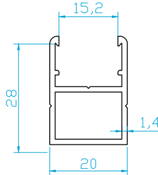
K2303 20x28 DEKO PROFIL (0.360 Kg/m)
