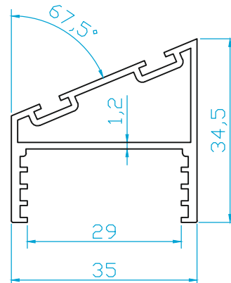
K4989 CAM BALKON KATLANIR SİSTEM 135° KÖŞE DÖNÜŞ (0.520 Kg/m)
