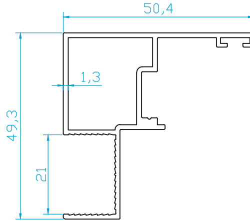
K1273 SPANYOLET KANAT 0.625 Kg/m
