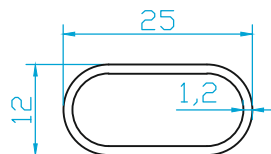
K238 DEKOR 0.195 Kg/m
