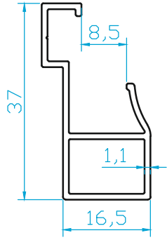
K1284 TABAN PROFİLİ 0.305 Kg/m
