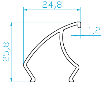
K2435 BALKON ÇİTA 0.225 Kg/m
