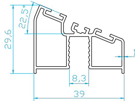
K1974 KARE TEKCAM AÇILI KANAT KENARI (22.5°) (MIKNATIS KANALLI) 0.490 Kg/m
