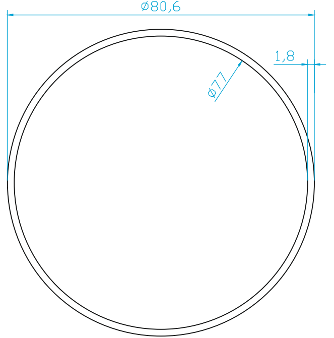
K276 Ø80 BORU (1.210 Kg/m)
