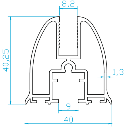
K4518 ÖZEL KANAT (0.810 Kg/m)
