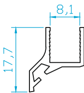
K4530 CAM FİTİL 0.143 Kg/m
