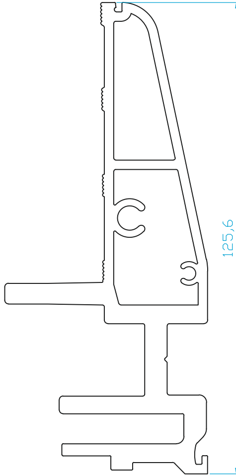
K1896 BALKON & PARAPET ŞASE 3.720 Kg/m
