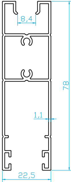
K5162 TEKCAM (8mm) BAZA 0.772 Kg/m
