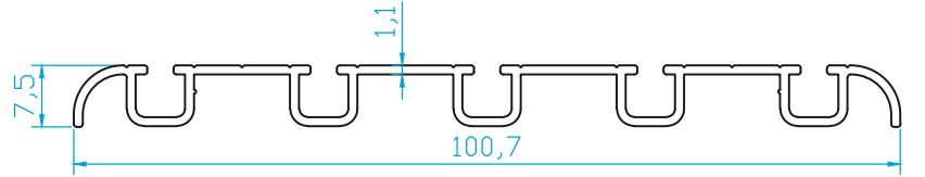
K4470 EŞİKSİZ ALT KASA 0.540 Kg/m
