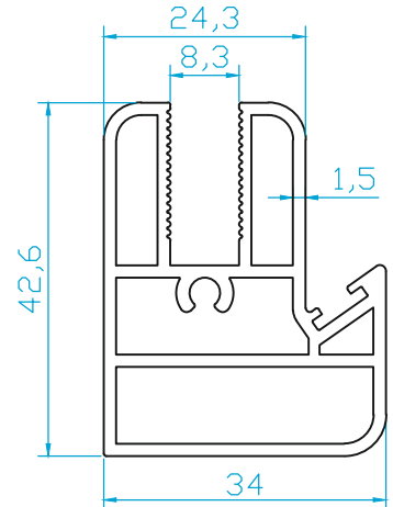
K1582 FİTİLLİ TEKCAM TUTUCU ARA PERDELİ 1.015 Kg/m
