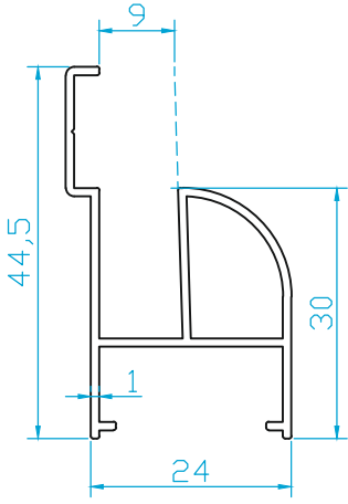
K2394 EKO TABAN PROFİLİ 0.360 Kg/m
