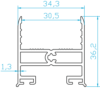
K1309 ISICAMBALKON KANAT (0.657 Kg/m)
