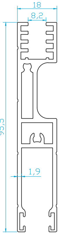
K4456 (8 mm CAM) SÜRME ALT KANAT 1.385 Kg/m
