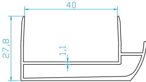
K4594 GEÇME DAMLALIK (0.560 Kg/m)
