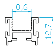
K4496 ÜST FİTİL 0.165 Kg/m
