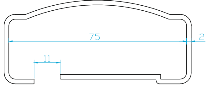
K2258 KÜPEŞTE BALKON AKSESUAR PRF. 1.060 Kg/m (K2257 için)
