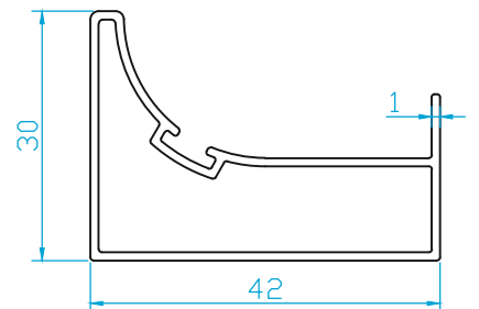
K4450 DiKME PROFİLİ (0.400 Kg/m)
