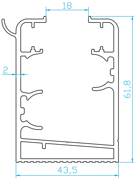
K4242 ÜSTTEN DAMLALIKLI KASA 1.350 Kg/m
