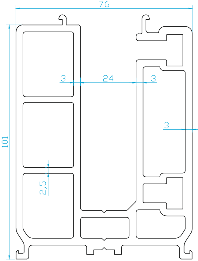
K1509 BALKON & PARAPET ŞASE (5.140 Kg/m)
