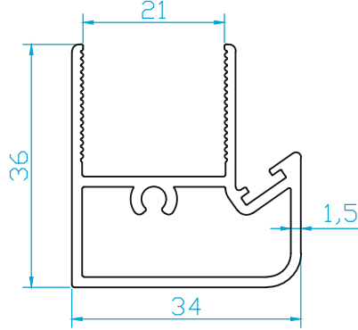
K1579 FİTİLLİ ÇİFTCAM TUTUCU KISA 0.645 Kg/m
