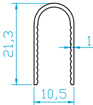
K1887 U PROFİL 0.130 Kg/m
