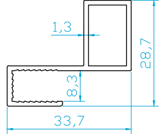
K1617 SPANYOLET KANAT 0.370 Kg/m
