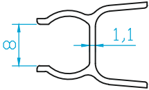
K4441 FİTİL PROFİLİ 0.166 Kg/m
