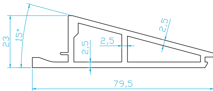
K1507 BALKON & PARAPET CAM AYAR PROFİLİ (1.250 Kg/m)
