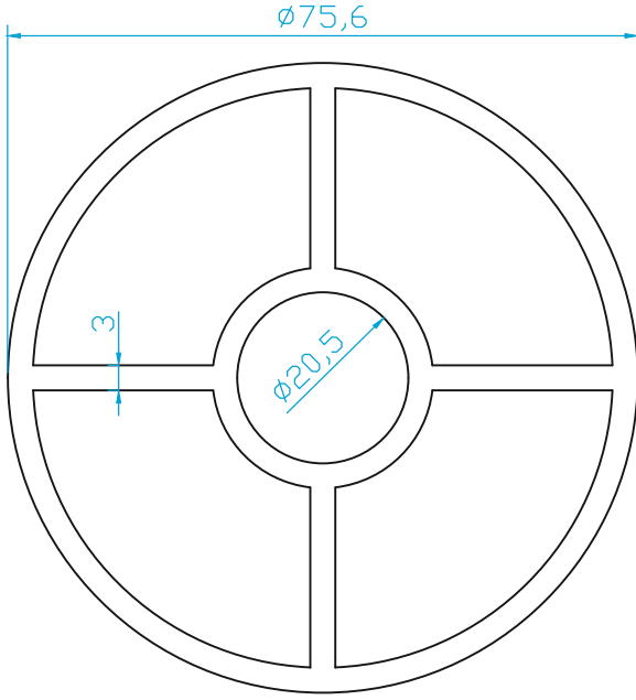
K277 DiKME (2.770 Kg/m)
