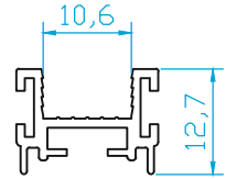
K4747 ÜST FİTİL 0.170 Kg/m
