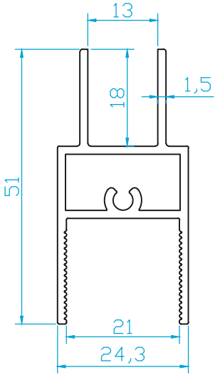
K4965 ÇİFTCAM TUTUCU ZİNCİR ASKILI (0.640 Kg/m)
