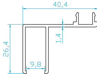
K268 CAM TUTUCU (8mm) 0.395 Kg/m
