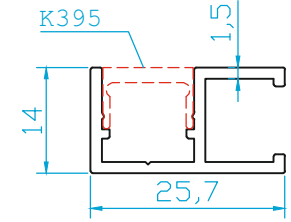
K396 CAM TUTUCU (0.270 Kg/m)
