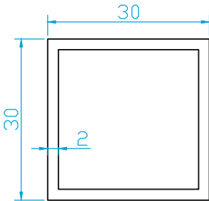
(K638) 30X30 (0.610 Kg/m)
