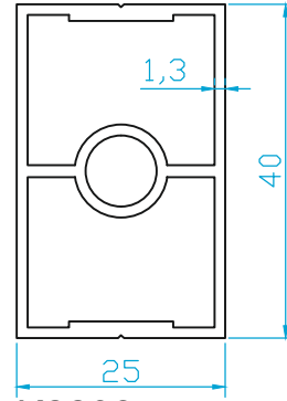
K2208 25X40 DİKME 0.650 Kg/m
