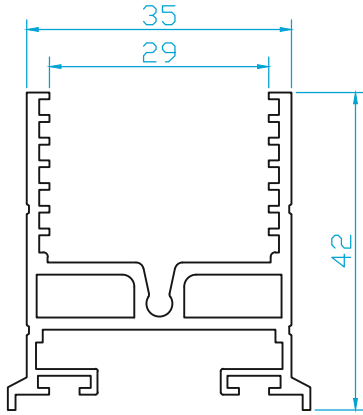
K4635 ÇİFTCAM KANAT (0.810 Kg/m)
