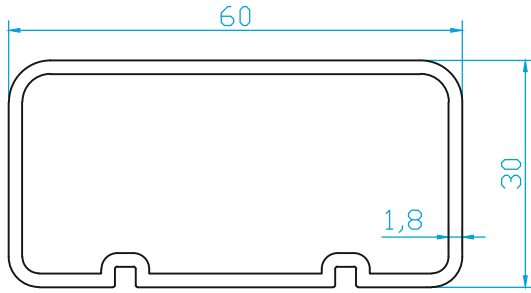
K251 KÜPEŞTE KORKULUK (0.850 Kg/m)
