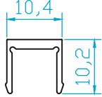
K236 40x40 DİKME KAPAK (K235 & K246 İÇİN) (0.095 Kg/m)
