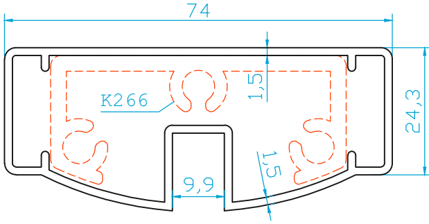
K2277 KÜPEŞTE BALKON PROFİLİ (0.950 Kg/m)
