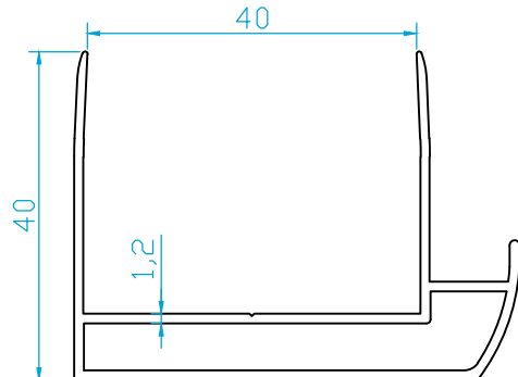
K4856 GEÇME DAMLALIK (0.600 Kg/m)
