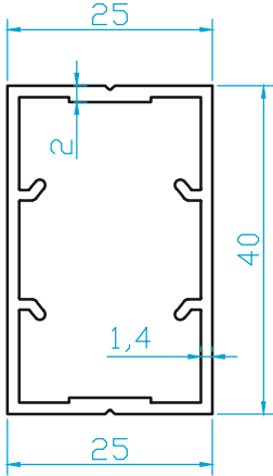
K2424 25X40 DİKME 0.570 Kg/m
