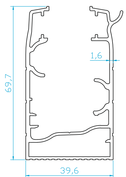
K4387 DAMLALIKLI KASA 1.200 Kg/m
