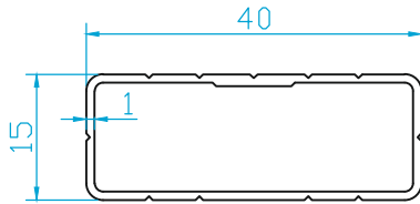
K2302 40x15 DEKO KUTU (0.290 kg/m)
