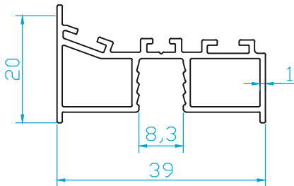
K1973 KARE TEKCAM KANAT KENARI (MIKNATIS KANALLI) 0.420 Kg/m
