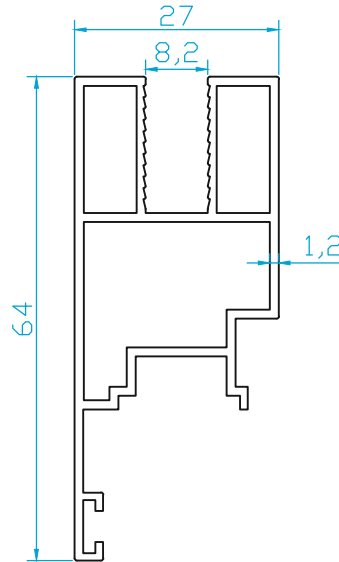
K1893 SPANYOLET KANAT 0.725 Kg/m
