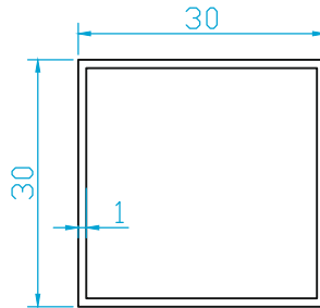
(K638) 30X30 (0.315 Kg/m)
