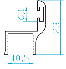
K4480 10 mm CAM FİTİL 0.185 Kg/m
