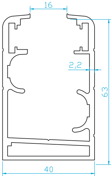
K4458 KASA (1.500 Kg/m)
