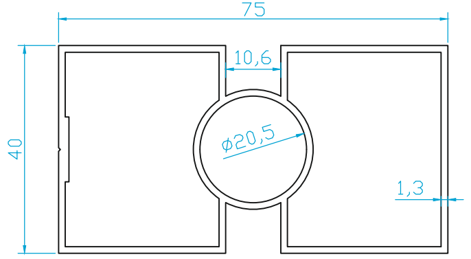
K2204 KÜPEŞTE DİKME PRF. (1.120 Kg/m)
