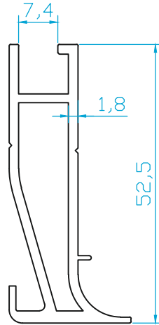
K4492 CAM TUTUCU (0.700 Kg/m)
