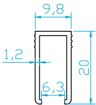
K250 CAM TUTUCU (6mm) 0.155 Kg/m
