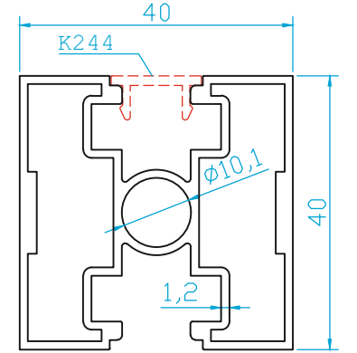
K269 KÜPEŞTE DİKME (0.965 Kg/m)
