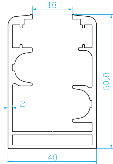
K4481 KASA (1.400 Kg/m)
