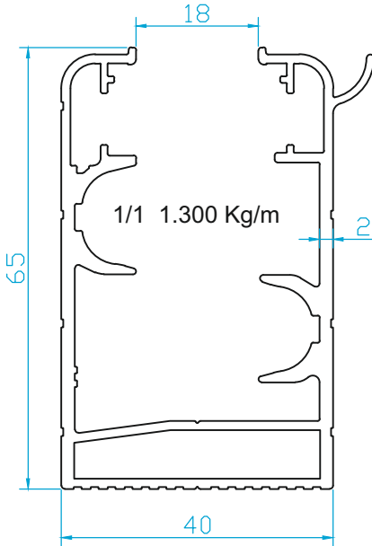
K4182 B KASA PROFİLİ 1.300 Kg/m
