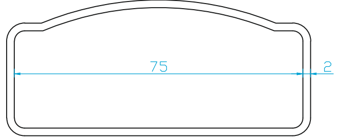
K2395 KÜPEŞTE BALKON AKSESUAR PRF. 1.125 Kg/m (K2390 için)
