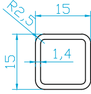
(K257) 15X15 (0.195 Kg/m)
