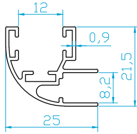
K4522 8mm CAM KÖŞE DÖNÜŞ 0.260 Kg/m
