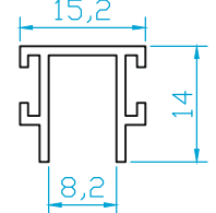
K4497 CAM TUTUCU 0.157 Kg/m
