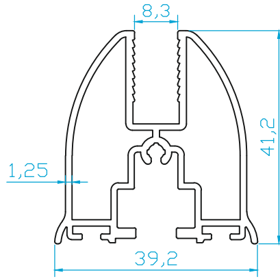
K1736 CAMBALKON KANAT 0.835 Kg/m
