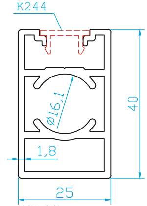
K243 25X40 DİKME 0.830 Kg/m
