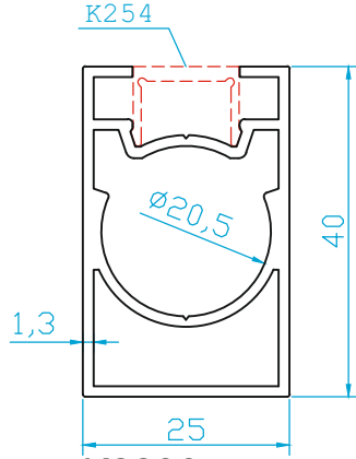
K2286 25X40 DİKME 0.660 Kg/m
