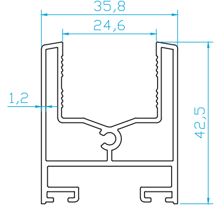
K1668 ÇİFTCAM KATLANIR KANAT (BKS TEKER) (0.800 Kg/m)
