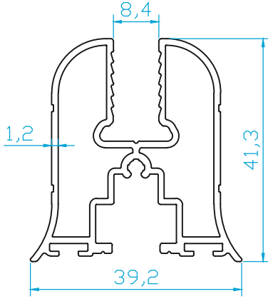
K4272 BAZA PROFİLİ 0.765 Kg/m
