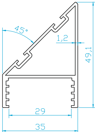
K4988 CAM BALKON KATLANIR SİSTEM 90° KÖŞE DÖNÜŞ (0.590 Kg/m)
