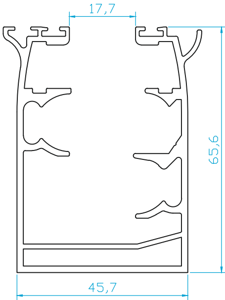
K1714 CAMBALKON KASA 1.538 Kg/m
