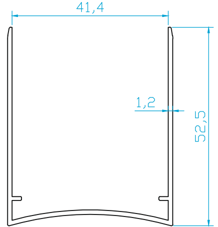
K2391 SEVİYE AYAR PROFİLİ (0.500 Kg/m) (ÜSTÜ OVAL KÜPEŞTELER için)
