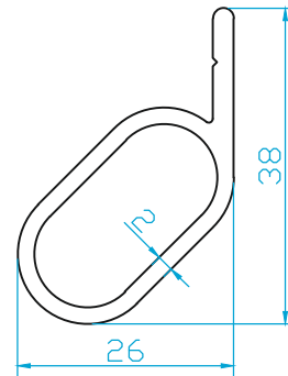
K2205 DEKOR PROFİLİ (0.500 Kg/m)
