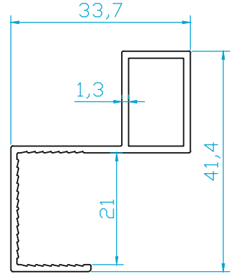
K1274 SPANYOLET KANAT 0.405 Kg/m
