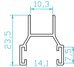
K4871 CAM FİTİL 10 mm 0.205 Kg/m
