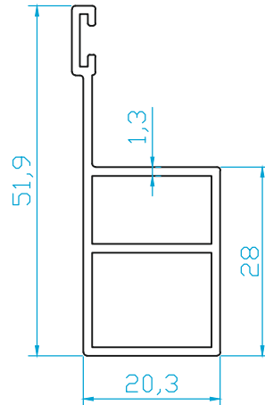
K6757 DiKME (0.495 Kg/m)
