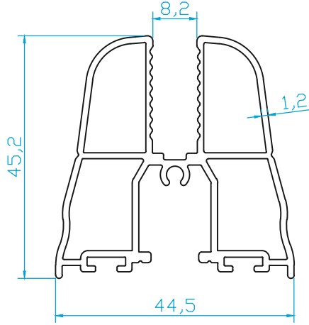
K4274 BAZA PROFİLİ 0.900 Kg/m
