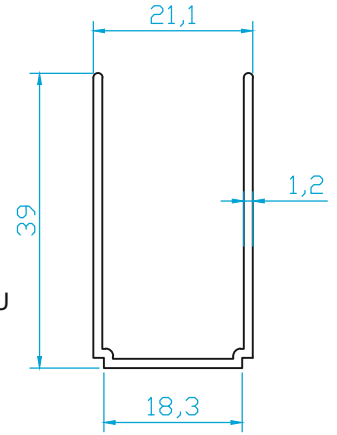
K4561 SÜRME FİX YAN U (0.315 Kg/m)
