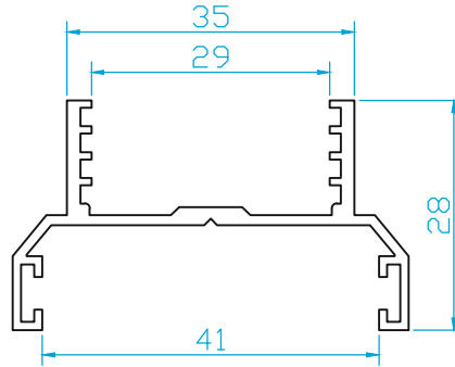
K4636 KANAT KARŞILIK (0.450 Kg/m)
