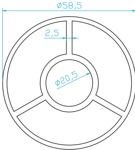
K278 DiKME (2.010 Kg/m)
