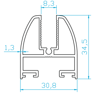
K1483 CAMBALKON KANAT 0.600 Kg/m
