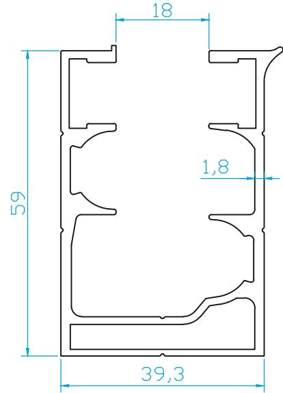
K1663 ÖZEL KASA (1.230 Kg/m)
