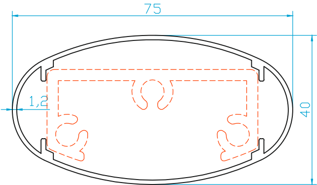
K2206 KÜPEŞTE BALKON PROFİLİ (0.700 Kg/m)
