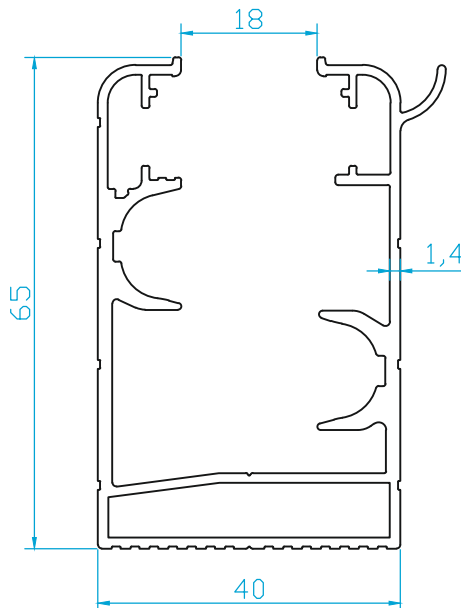
K4182 KASA PROFİLİ 1.250 Kg/m
