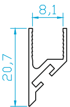
K4529 CAM FİTİL 0.145 Kg/m
