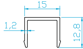
K2304 20x28 DEKO KAPAK 0.125 Kg/m
