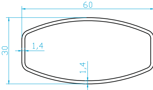
K2428 KÜPEŞTE PROFİLİ (0.585 Kg/m)
