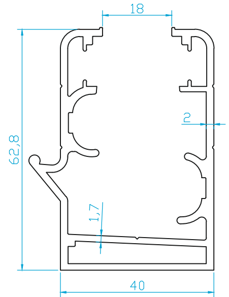
K4855 KASA (DAMLALIKLI) (1.430 Kg/m)
