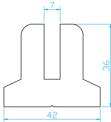
K2226 KÜPEŞTE AKSESUAR 2.570 Kg/m
