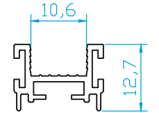
K4747 CAM KARŞILIK 10 mm 0.170 Kg/m
