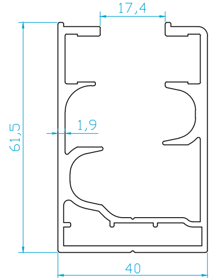
K1640 CAMBALKON KASA 1.385 Kg/m
