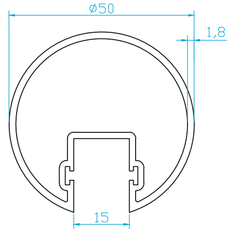
K7750 BALKON ÜST PROFİLİ (0.945 Kg/m)
