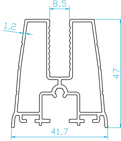
K4183 BAZA PROFİLİ 0.865 Kg/m
