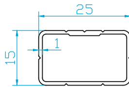
K2344 25x15 DEKO KUTU (0.208 Kg/m)
