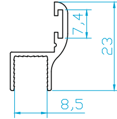
K4632 8mm CAM KARŞILIK (0.170 Kg/m)
