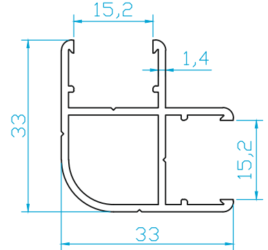
K2355 20x33 DEKO KÖŞE (0.500 Kg/m)
