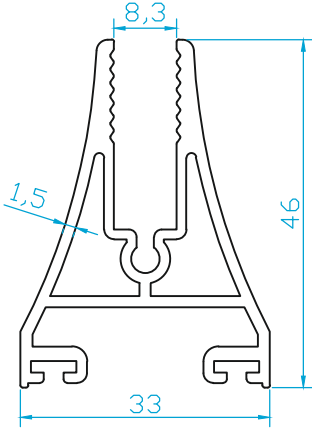
K1715 CAMBALKON KANAT 0.875 Kg/m
