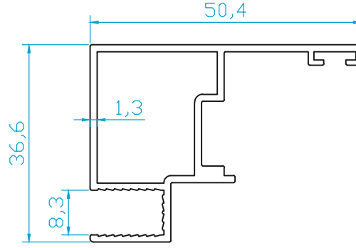
K1616 SPANYOLET KANAT 0.585 Kg/m
