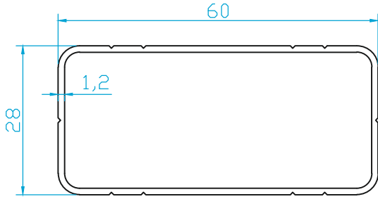
K2300 60x28 DEKO KUTU (0.540 Kg/m)
