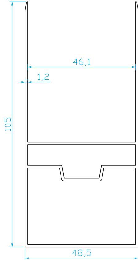
K4886 ÜST AYAR PROFİLİ 1.160 Kg/m
