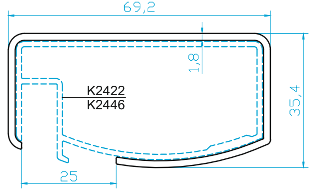
K2423 KÜPEŞTE BALKON AKSESUAR PRF. (0.805 Kg/m)
