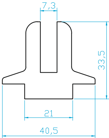
K2426 KÜPEŞTE AKSESUAR 1.620 Kg/m
