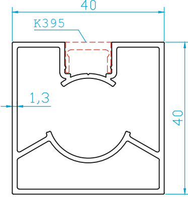
K384 KÜPEŞTE DİKME (0.830 Kg/m)
