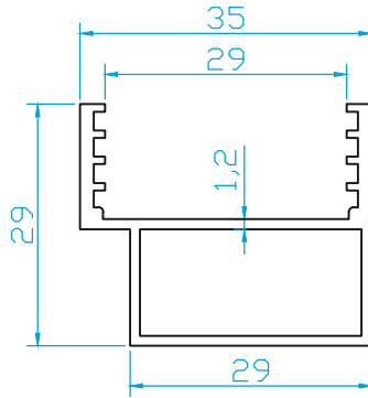
K4638 DİKME KARŞILIK (0.460 Kg/m)
