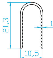
K1887 U PROFİL 0.130 Kg/m
