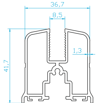
K4559 CAM BALKON KATLANIR KANAT (0.850 Kg/m)
