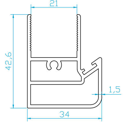
K1581 FİTİLLİ ÇİFTCAM TUTUCU ARA PERDELİ 0.840 Kg/m
