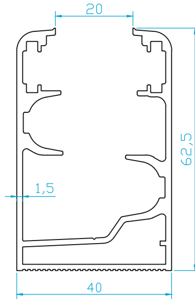
K1621 CAMBALKON KASA 1.215 Kg/m
