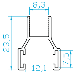
K4772 CAM FİTİL 0.195 Kg/m
