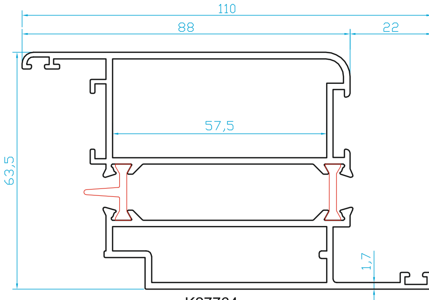
K27764 KAPI KANAT PROFİL (2.260 Kg/m)
