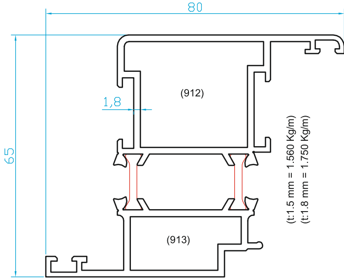
K2912 GENİŞ KANAT
