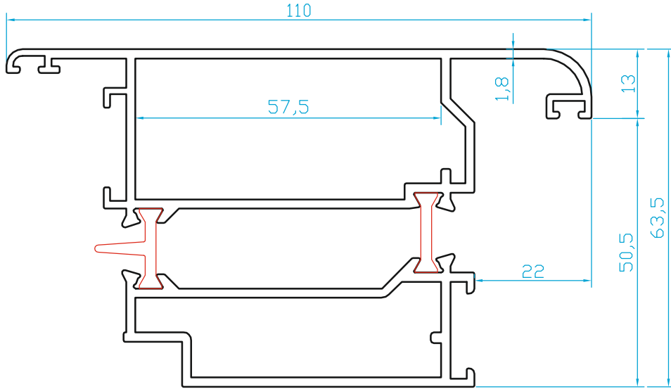
K27770 DIŞA AÇILIM KAPI KANAT PROFİL (2.350 Kg/m)
