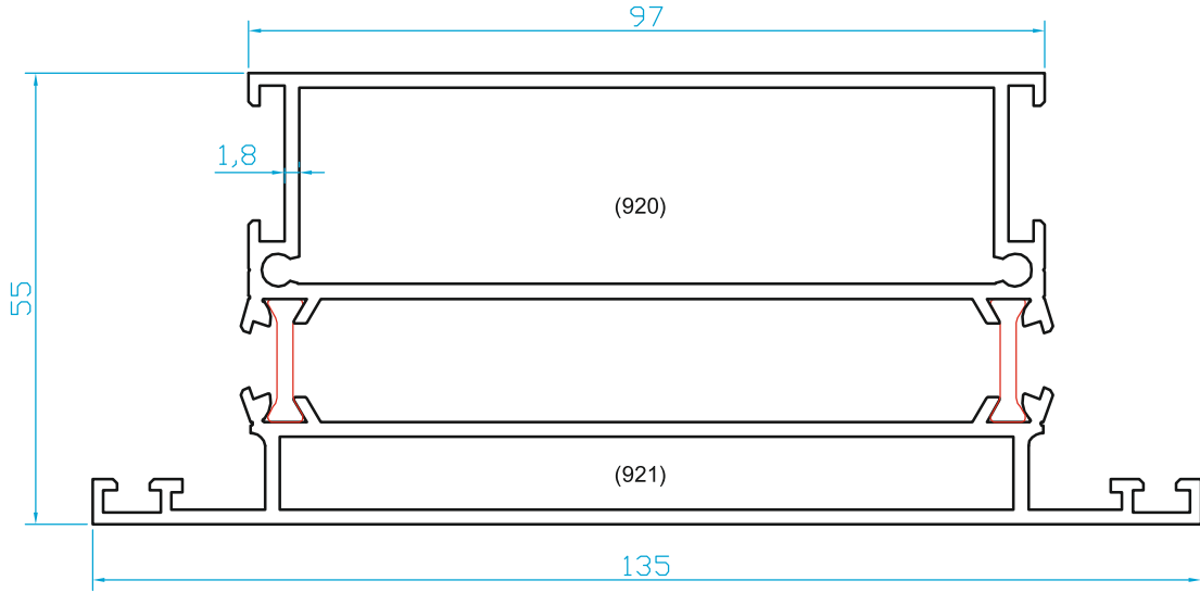
K2920 GENİŞ ORTA BAZA (2.900 Kg/m)
