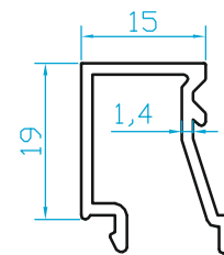
K990 ISI YALITIM ÇITA 6+16+6=28 mm CAM İÇİN 0.270 Kg/m
