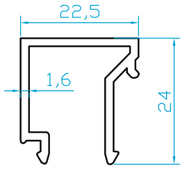
K961 ÇİFTCAM ÇITA (0.330 Kg/m)
