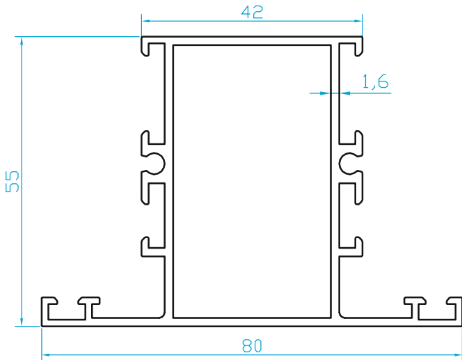
K400 ORTA KAYIT (1.250 Kg/m)
