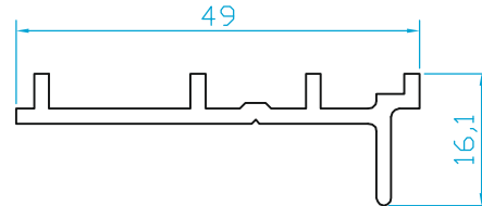
K412 KASA KANAT ADAPTÖRÜ (0.380 Kg/m)
