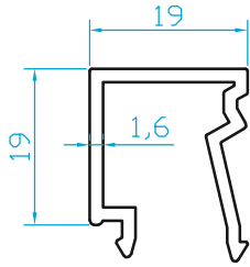
K2938 ISICAM FİTİLLİ ÇİTA (0.370 Kg/m)
