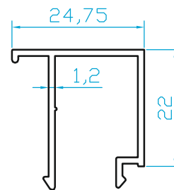
K8811 10mm TEKCAM ÇİTASI (0.260 Kg/m)
