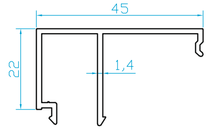
K837 ÇİTA (BİM-K808 VE K811'E) (0.395 Kg/m)
