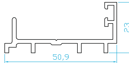
K411 KASA KANAT ADAPTÖRÜ (0.510 Kg/m)
