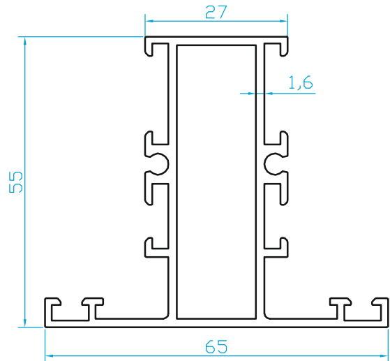
K431 DAR ORTA KAYIT (1.100 Kg/m)
