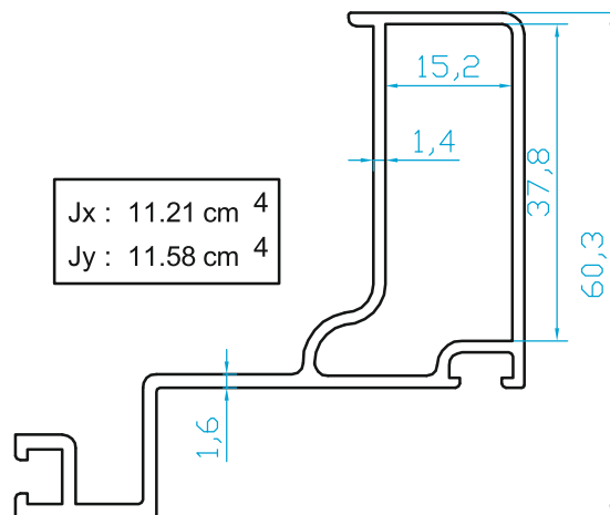
K4589 ALUNEW SERİ GİZLİ KANAT, KANAT PRF (0.885 Kg/m)
