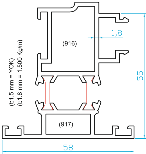
K2916 KANAT ADAPTÖRÜ
