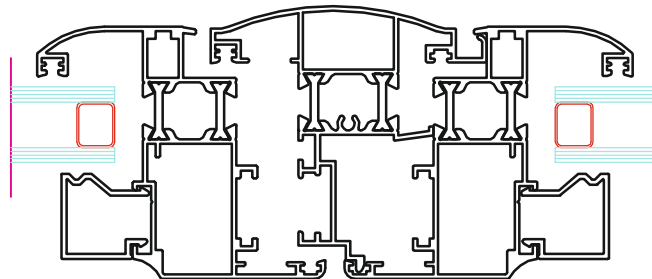
DAR KANAT-ADAPTÖR -ÇITA UYGULAMASI (ÖLÇEK/Scale:1/2)
