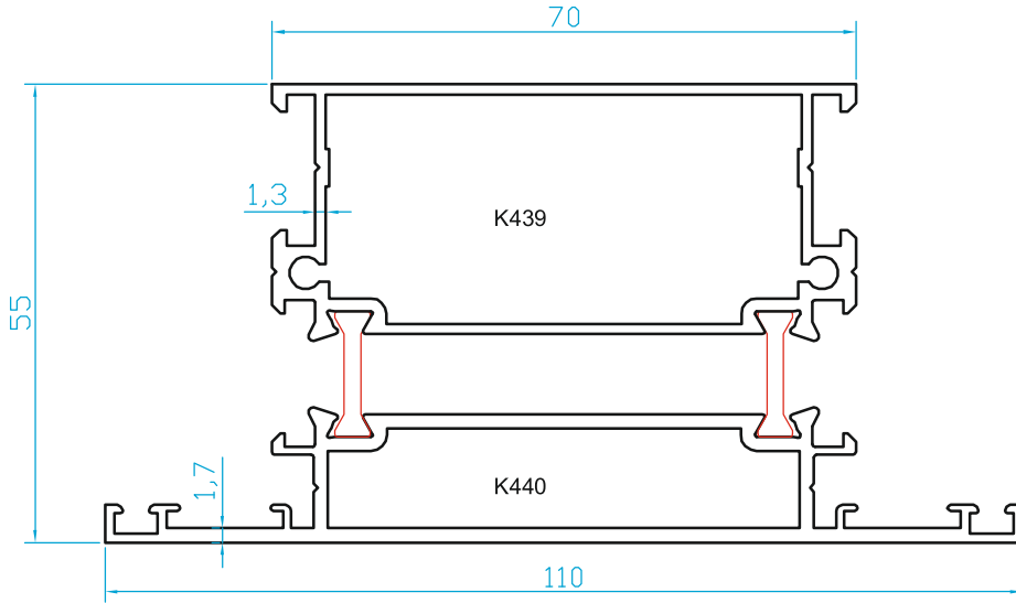
K2439 GENİŞ ORTA KAYIT (2.000 Kg/m)
