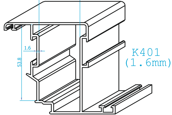
K401 (1.6 mm) KÖŞE TAKOZU UYGULAMASI
