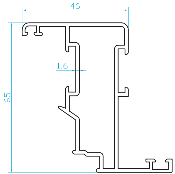
K433 DAR KANAT (1.100 Kg/m)
