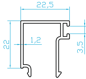
K7763 20 mm ÇİFTCAM ÇITA (0.275 Kg/m)
