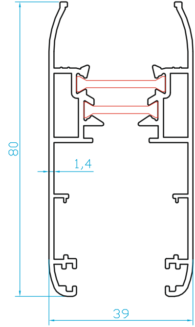
K27752 YALITIMLI SÜRME KANAT (1.300 Kg/m)
