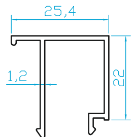
K812 TEKCAM ÇİTASI (0.265 Kg/m)
