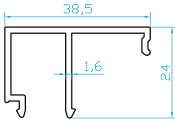
K960 TEKCAM ÇITA (0.400 Kg/m)
