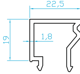
K2918 ISICAM ÇİTASI (t:1.3 mm = 0.265 Kg/m) (t:1.8 mm = 0.325 Kg/m)
