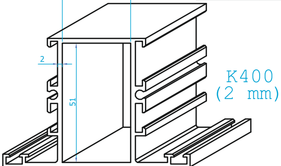
K400 (2 mm) KÖŞE TAKOZU UYGULAMASI
