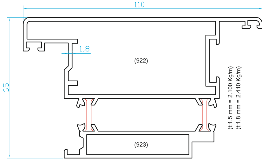
K2922 DIŞA AÇILAN KAPI
