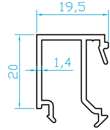
K2443 ÇITA (24 mm CAM) (0.295 Kg/m)
