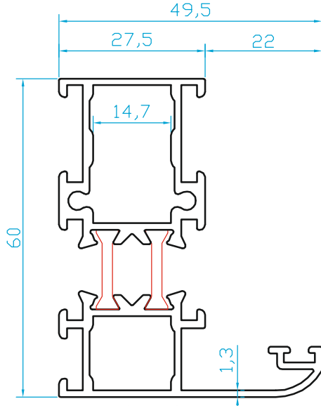
K27758 PENCERE KASA PROFİL (1.290 Kg/m)
