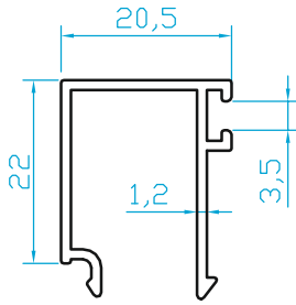
K7762 24 mm ÇİFTCAM ÇITA (0.265 Kg/m)
