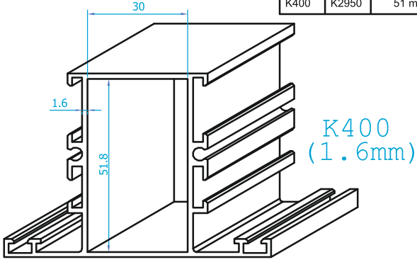
K400 (1.6mm) KÖŞE TAKOZU UYGULAMASI
