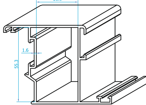
K403 (1.6mm) KÖŞE TAKOZU UYGULAMASI
