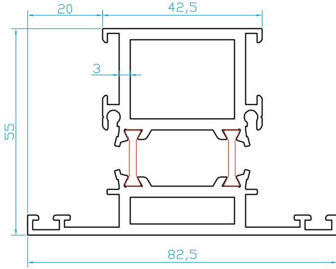
K2954 ORTA KAYIT (2.200 Kg/m)
