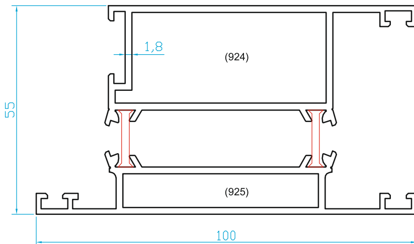
K2924 GENİŞ ETEK (2.160 Kg/m)
