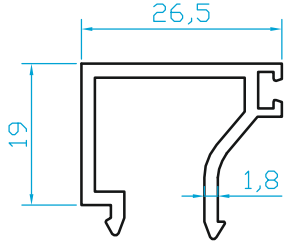
K2938 ISICAM FİTİLLİ ÇİTA (0.370 Kg/m)
