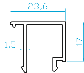
K815 ISICAM ÇİTASI (0.240 Kg/m)
