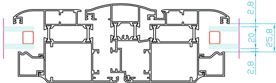
GENİŞ KANAT-ADAPTÖR -ÇITA UYGULAMASI (ÖLÇEK/Scale:1/2)
