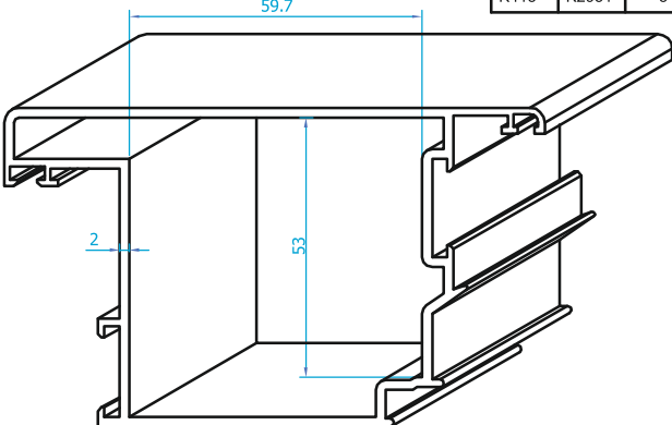
K413 (2 mm) KÖŞE TAKOZU UYGULAMASI
