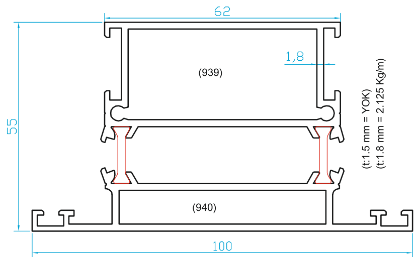
K2939 100'LÜK ORTA
