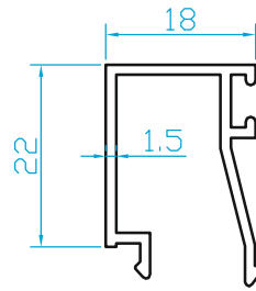
K816 FİTİLLİ CAM ÇİTASI (0.255 Kg/m) (18mm ÇİFTCAM)
