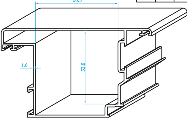
K413 (1.6mm) KÖŞE TAKOZU UYGULAMASI
