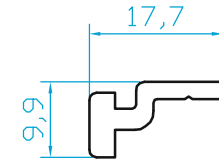
K4585 ALUNEW SERİ KASET MONTAJ PRF. (0.190 Kg/m)
