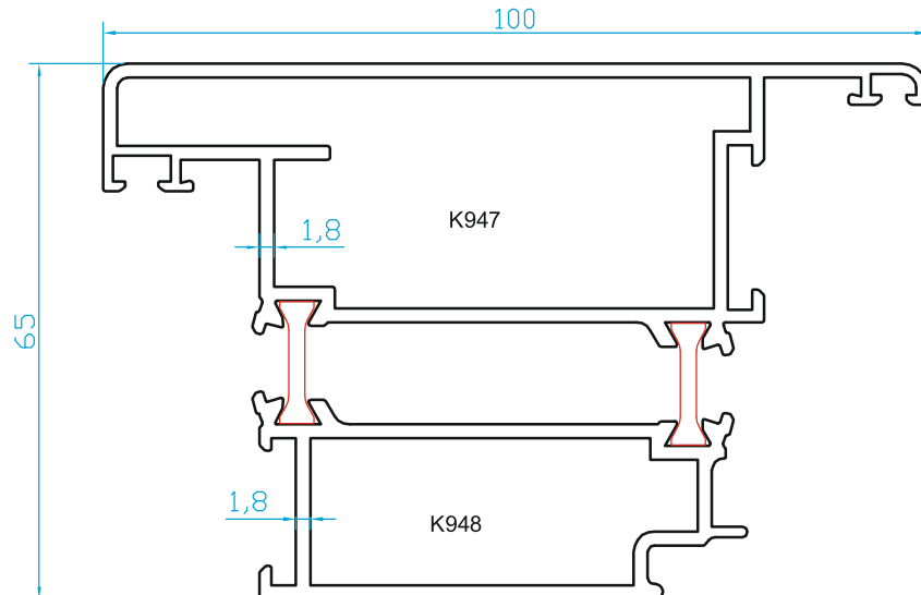
K2947 100'LÜK DIŞA AÇILIM KAPI KANAT (2.100 Kg/m)
