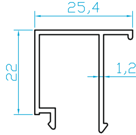
K812 8 mm TEKCAM ÇİTASI (0.270 Kg/m)
