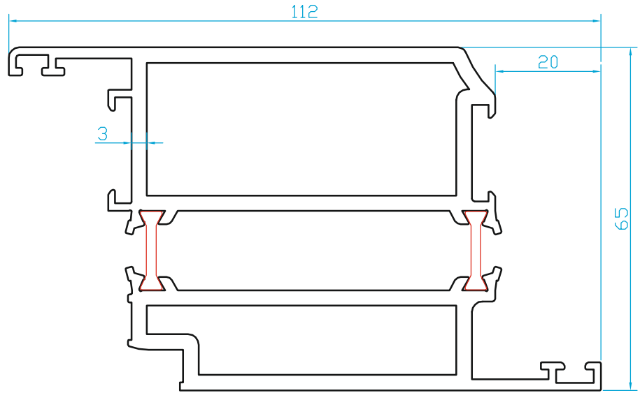
K2958 KAPI KANAT (3.300 Kg/m)
