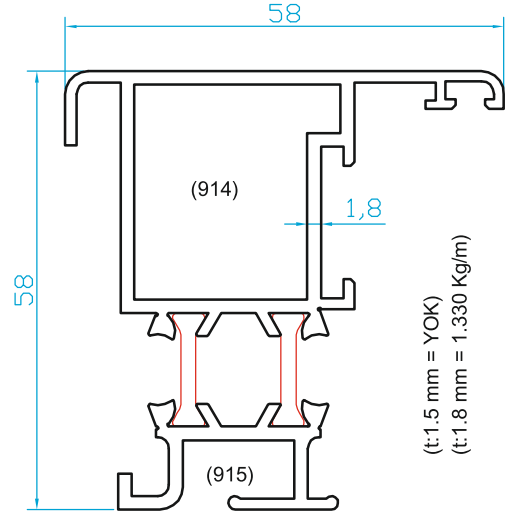
K2914 PİVOT ADAPTÖRÜ
