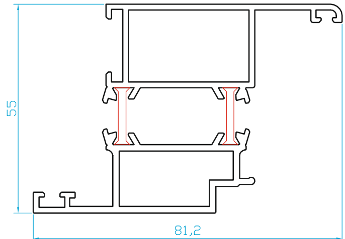
K2966 (1.350 Kg/m) ÖZEL PERVAZLI KASA
