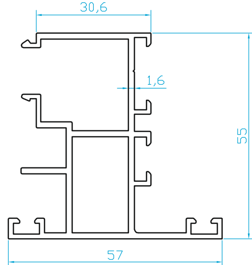
K434 KANAT PİVOT ADAPTÖRÜ (ÖZEL) (1.070 Kg/m)
