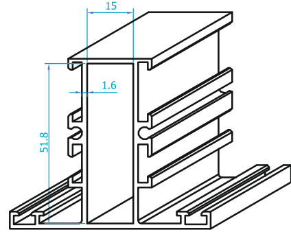
K431 (1.6mm) KÖŞE TAKOZU UYGULAMASI
