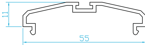
K404 ÇARPMA KAPI ADAPTÖRÜ (0.370 Kg/m)
