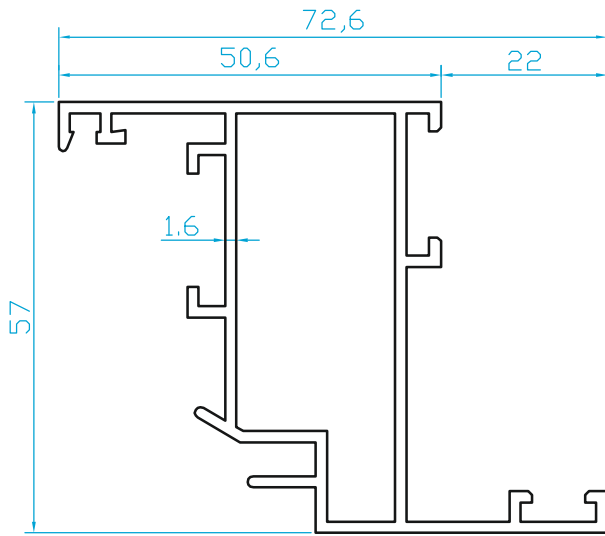
K803 C50 DAR KANAT (1.090 Kg/m)
