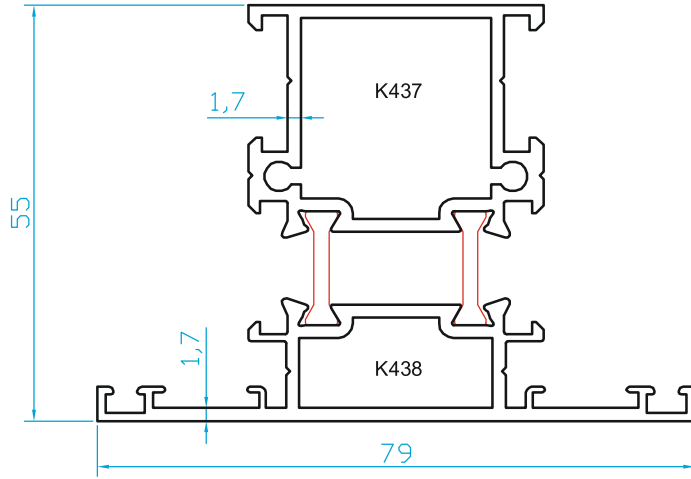
K2437 ORTA KAYIT (1.600 Kg/m)
