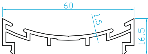
K819 ÇARPMA KAPI KASA ADAPTÖRÜ (0.445 Kg/m)
