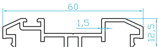
K822 ÇARPMA KAPI KASA ADAPTÖRÜ (0.440 Kg/m)
