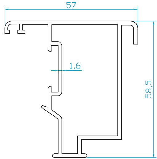
K408 KASA PİVOT ADAPTÖRÜ (1.000 Kg/m)
