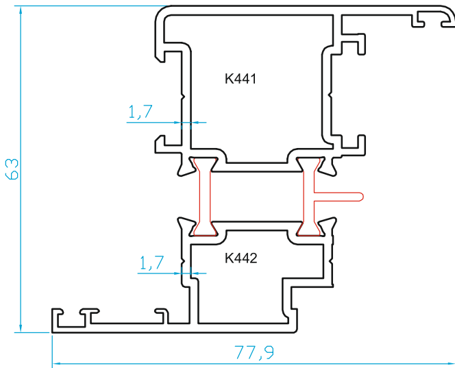
K2441 KANAT (1.650 Kg/m)
