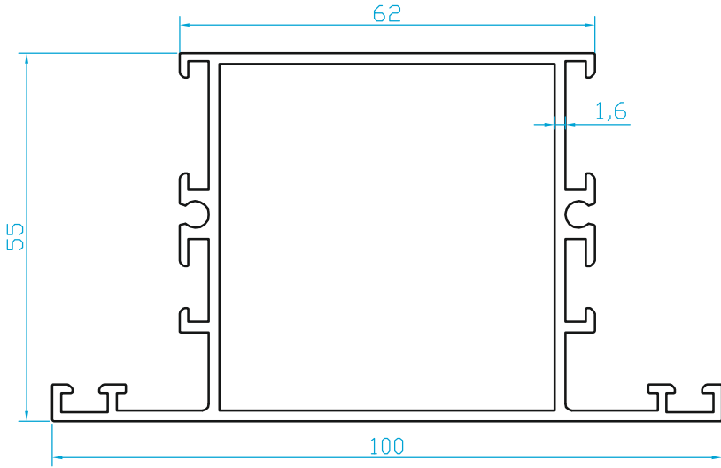
K414 GENİŞ ORTA KAYIT (1.430 Kg/m)
