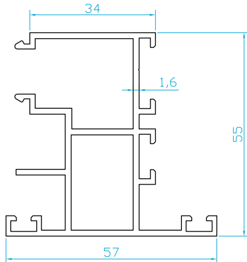
K407 KANAT PİVOT ADAPTÖRÜ (1.100 Kg/m)
