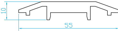
K405 ÇARPMA MENTESE ALT TAKOZU (0.670 Kg/m)
