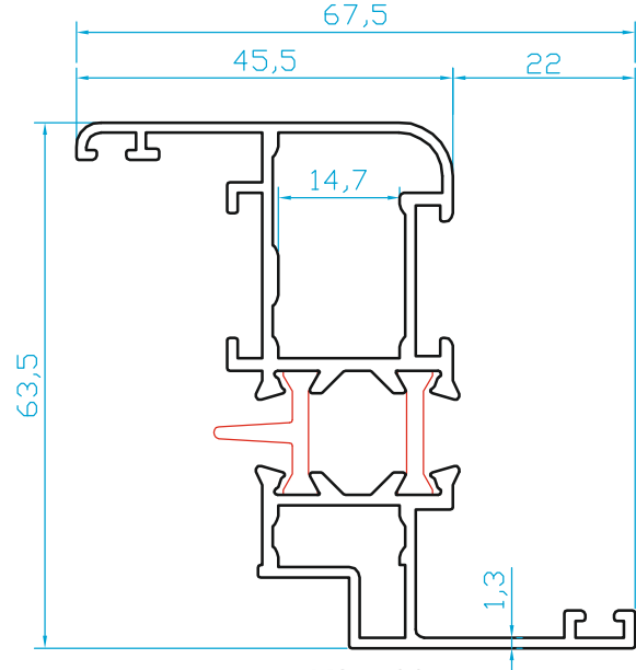
K27760 PENCERE KANAT PROFİL (1.270 Kg/m)
