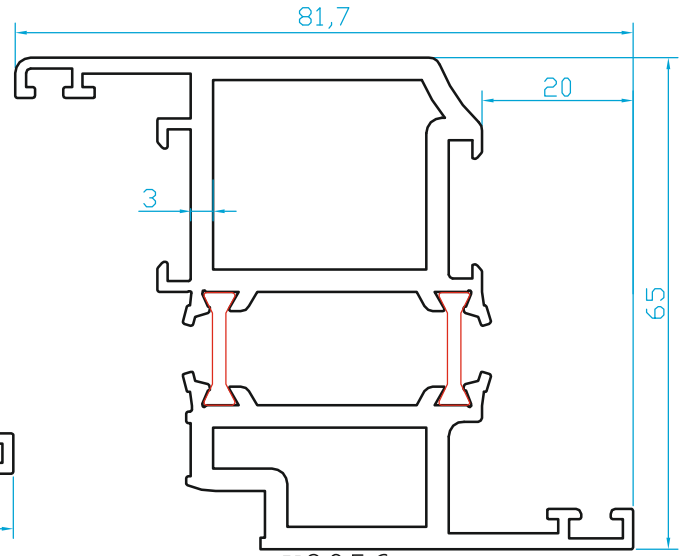
K2956 NORMAL KANAT (2.350 Kg/m)
