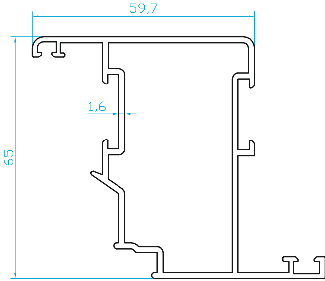
K401 GENİŞ KANAT (1.240 Kg/m)
