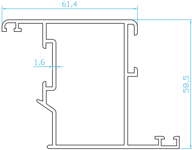
K403 KANAT (1.190 Kg/m)
