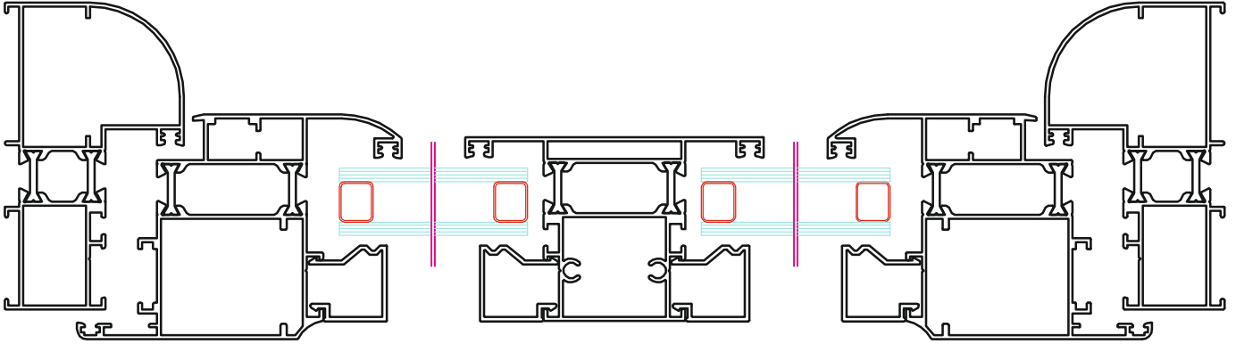
KASA-GENİŞ KANAT-KAYIT -ÇITA UYGULAMASI (ÖLÇEK/Scale:1/2)
