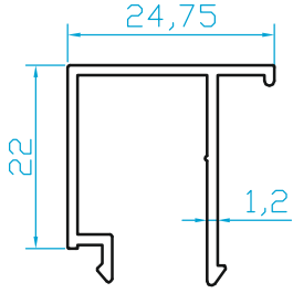
K8811 10 mm TEKCAM ÇİTASI (0.265 Kg/m)
