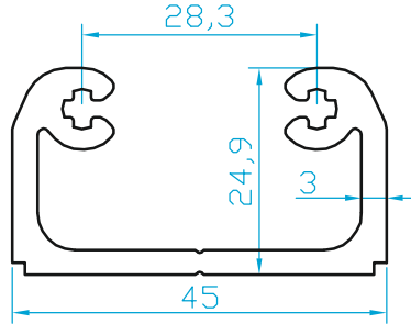
K4628 CEPHE KAYIT BAĞLANTI 0.990 Kg/m
