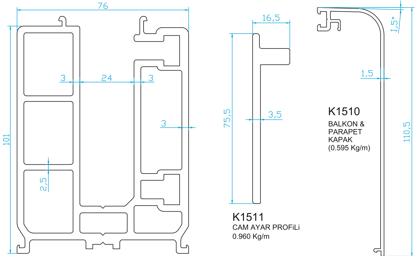
K1509 BALKON & PARAPET ŞASE (5.140 Kg/m)
