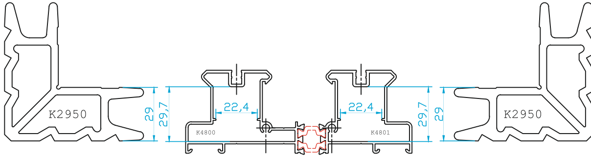
K24800 KALDIR SÜR KASA KÖŞE TAKOZU UYGULAMASI (ÖLÇEK 1/2)
