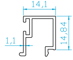
K540 ÇITA (0.190 Kg/m)
