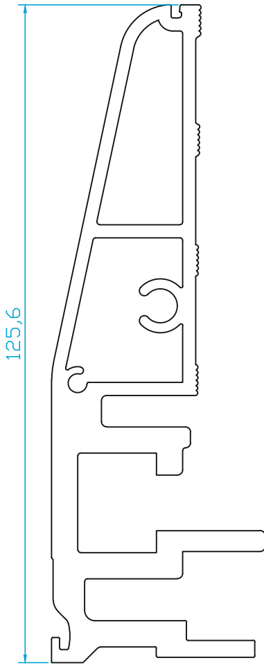
K1895 BALKON & PARAPET ŞASE 3.560 Kg/m
