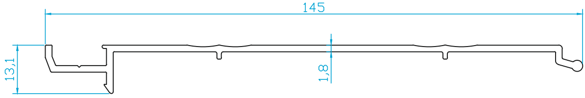
K5361 MOTOR KUTUSU KAPAK (0.800 Kg/m)
