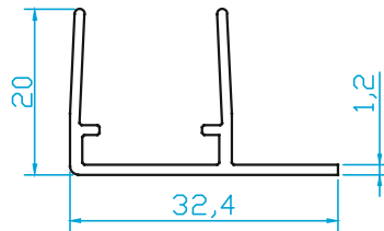
K1345 Kondensprofil 0.249 Kg/m
