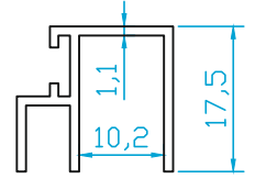
K4495 CAM TUTUCU 10 mm 0.200 Kg/m
