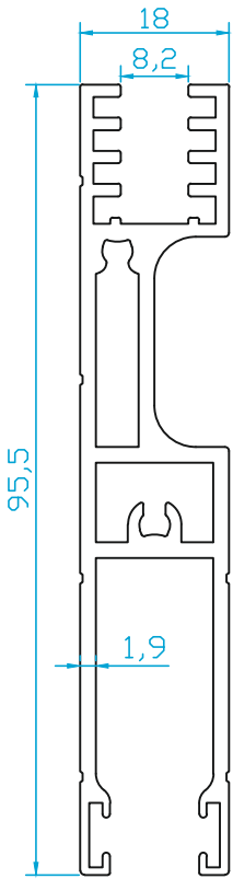
K4456 (8 mm CAM) SÜRME ALT KANAT 1.385 Kg/m
