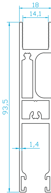
K4537 SÜRME ALT KANAT 1.110 Kg/m
