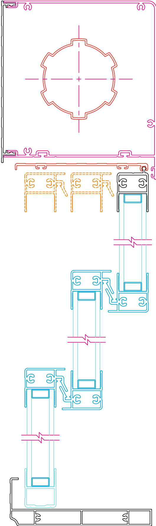
C-C KESİTİ GIYOTİN SİSTEM KAPALI KESİT (DİKEY)
