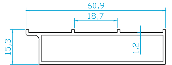
K4599 SÜRME FİX YAN KASA 0.460 Kg/m
