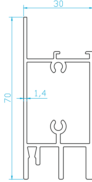
K327 FOTOSEL KAPI ETEK (1.050 Kg/m)
