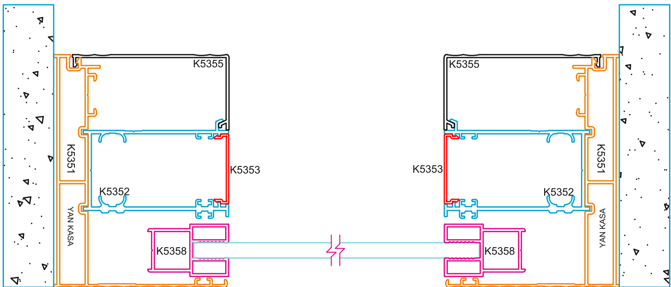
B-B KESİTİ GİYOTİN SİSTEM KAPALI KESİT (YATAY)
