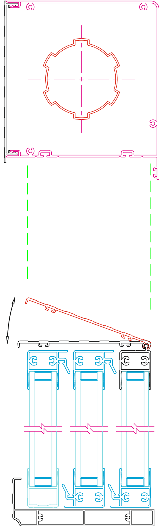
D-D KESİTİ GIYOTİN SİSTEM AÇIK KESİT (DİKEY)
