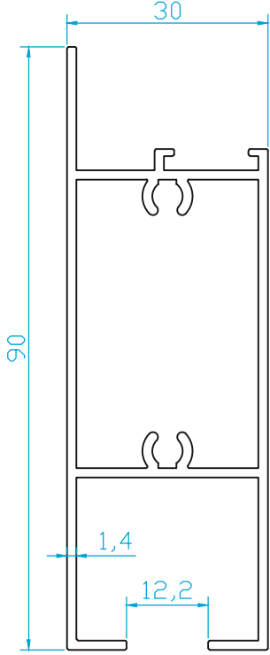
K6733 FOTOSEL KAPI KANAT (0.998 Kg/m)
