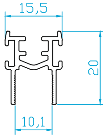
K1853 CAM ÜST FİTİLİ (0.217 Kg/m)
