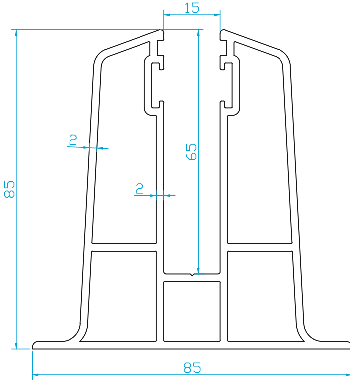
K2305 BALKON TABAN PROFİLİ (2.730 Kg/m)
