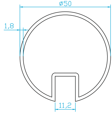
K2250 BALKON ÜST PROFİLİ 0.870 Kg/m
