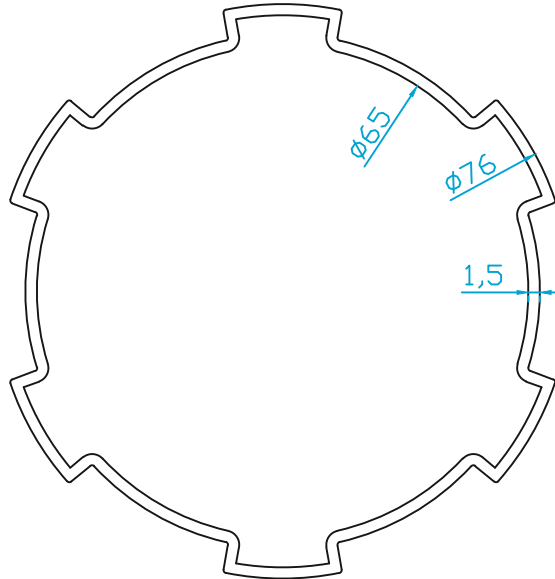
K5478 TENTE MOTOR BORUSU PROFİLİ 1.075 Kg/m
