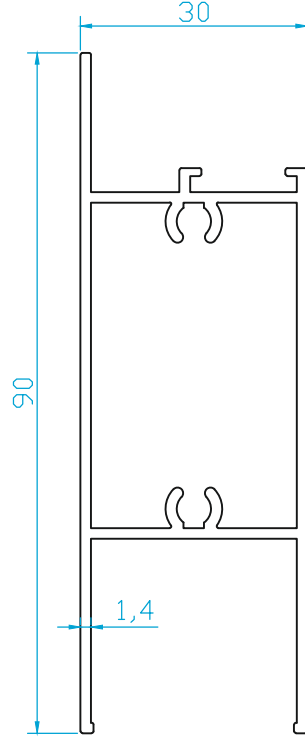
K6734 FOTOSEL KAPI KANAT (0.945 Kg/m)
