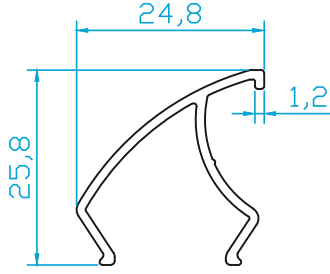
K2435 BALKON ÇİTA 0.225 Kg/m
