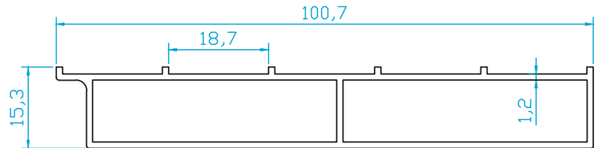
K4560 SÜRME FİX YAN KASA 0.770 Kg/m
