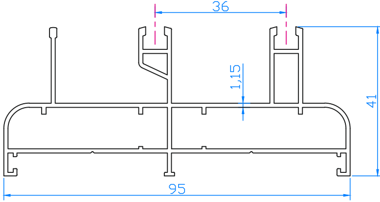
K1687 YALITIMSIZ SÜRME KASA 95 36 mm AKS (1.180 Kg/m)
