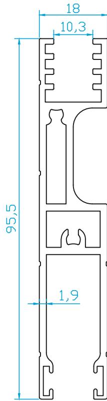
K4498 (10 mm CAM) SÜRME ALT KANAT 1.340 Kg/m
