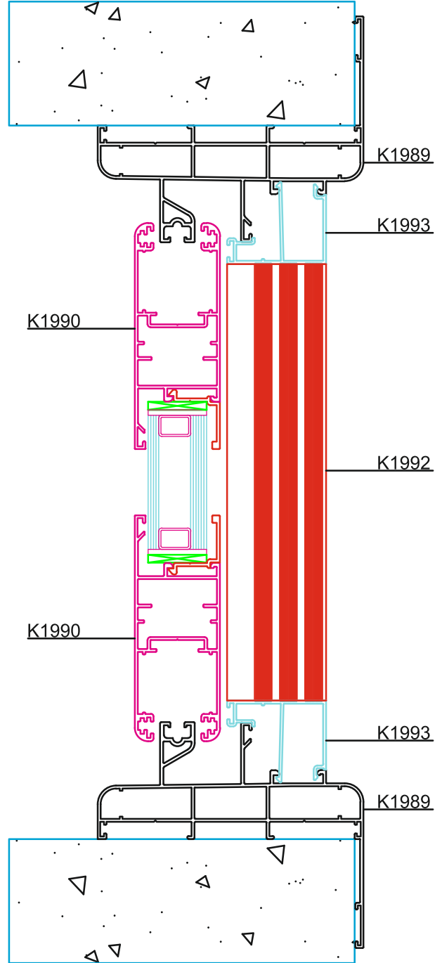
B-B KESİTİ
