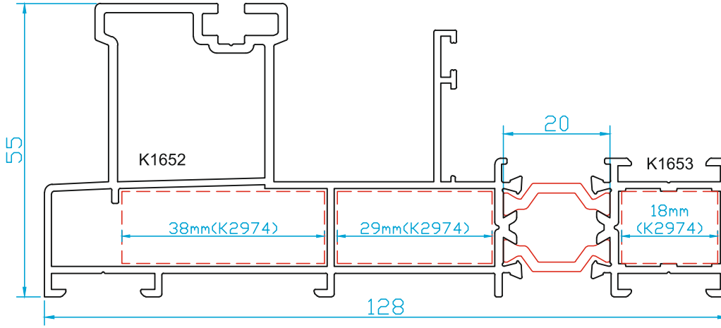
K21652 KALDIR SÜR KASA TKM SiP. NR: K21652 2.410 Kg/m (ISI BARIYERLi)
