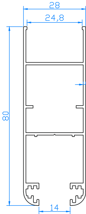
K1673 28x80 SÜRME KANAT ÇİFTCAM (0.790 Kg/m)
