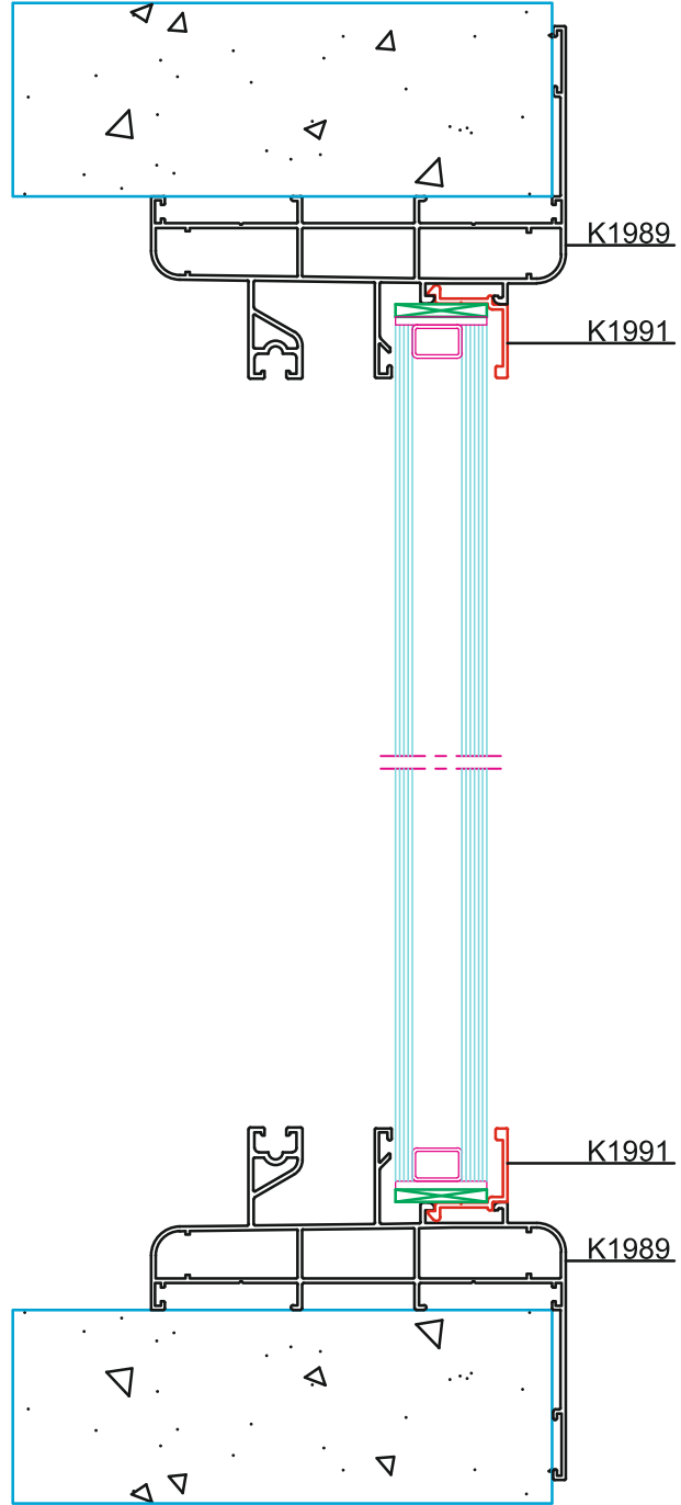
C-C KESİTİ
