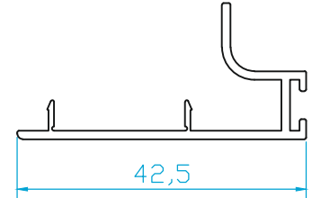
K6736 KENET KAPAK (0.265 Kg/m)
