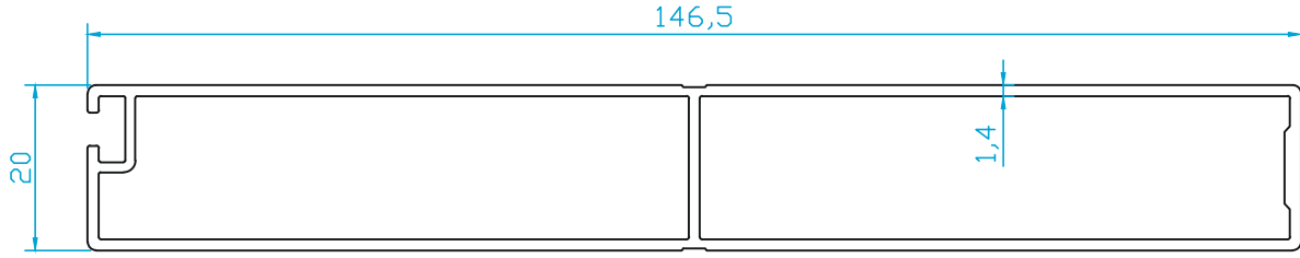
K5472 TENTE ARA KAYIT PROFİLİ (1.580 Kg/m)
