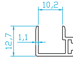
K5233 10 MM CAM TUTUCU 0.138 Kg/m
