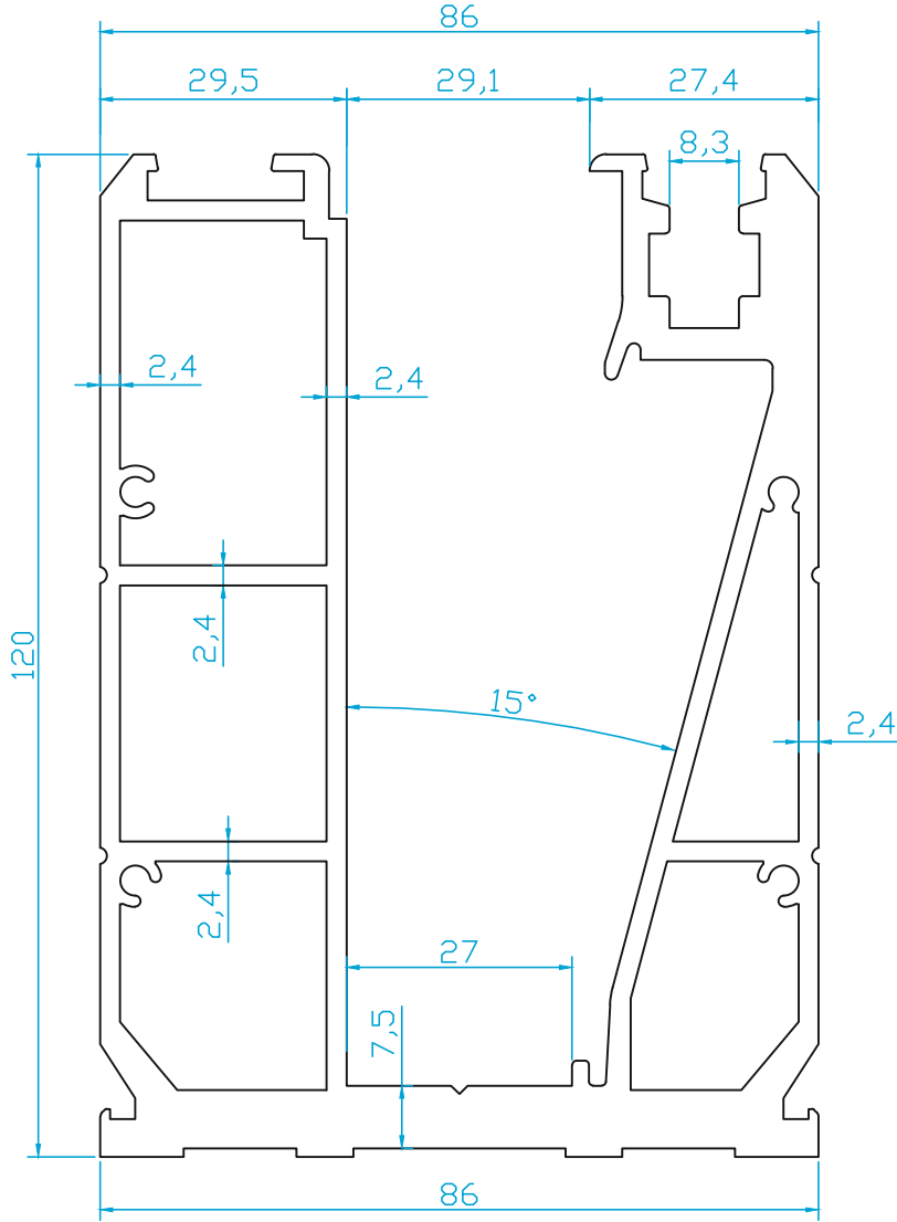
K1506 BALKON & PARAPET ŞASE (6.420 Kg/m)
