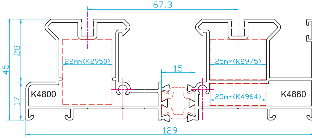
K24860 KALDIR SÜR KASA TKM SİP. NR: K24860 2.300 Kg/m (ISI BARIYERLİ)
