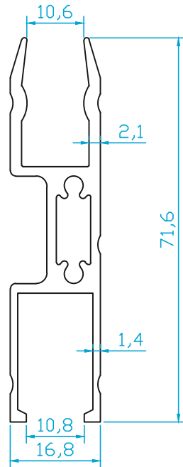
K5234 SÜRME KANAT 0.910 Kg/m
