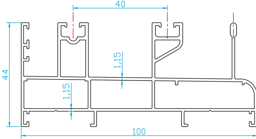
K1669 YALITIMSIZ SÜRME KASA (1.520 Kg/m)
