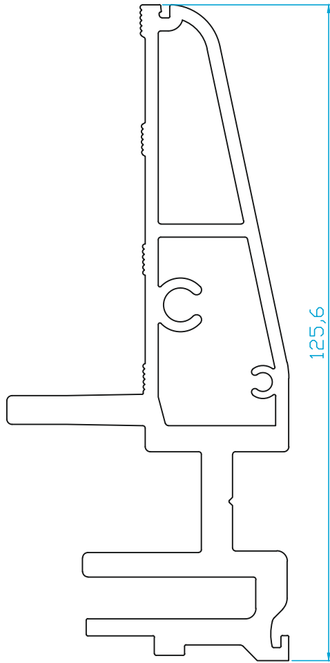
K1896 BALKON & PARAPET ŞASE 3.720 Kg/m
