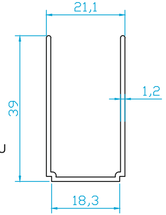
K4470 EŞİKSİZ ALT KASA 0.540 Kg/m
