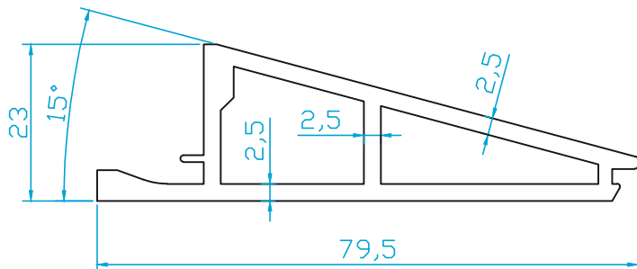
K1507 BALKON & PARAPET CAM AYAR PROFİLİ (1.250 Kg/m)
