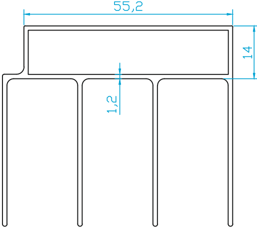
K4460 SÜRME ÜST KASA (3LÜ) 0.950 Kg/m
