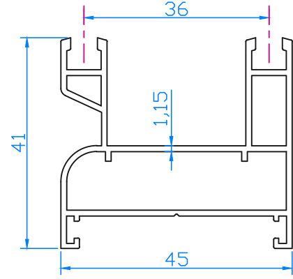
K1689 YALITIMSIZ SÜRME KASA 45 36 mm AKS (0.735 Kg/m)
