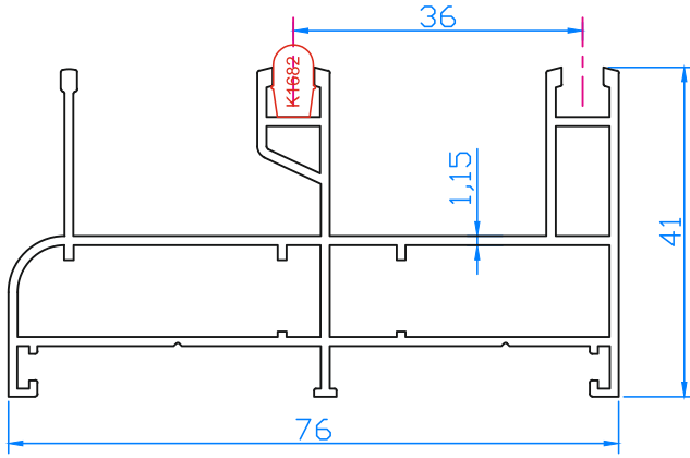
K1688 YALITIMSIZ SÜRME KASA 76 36 mm AKS (1.065 Kg/m)
