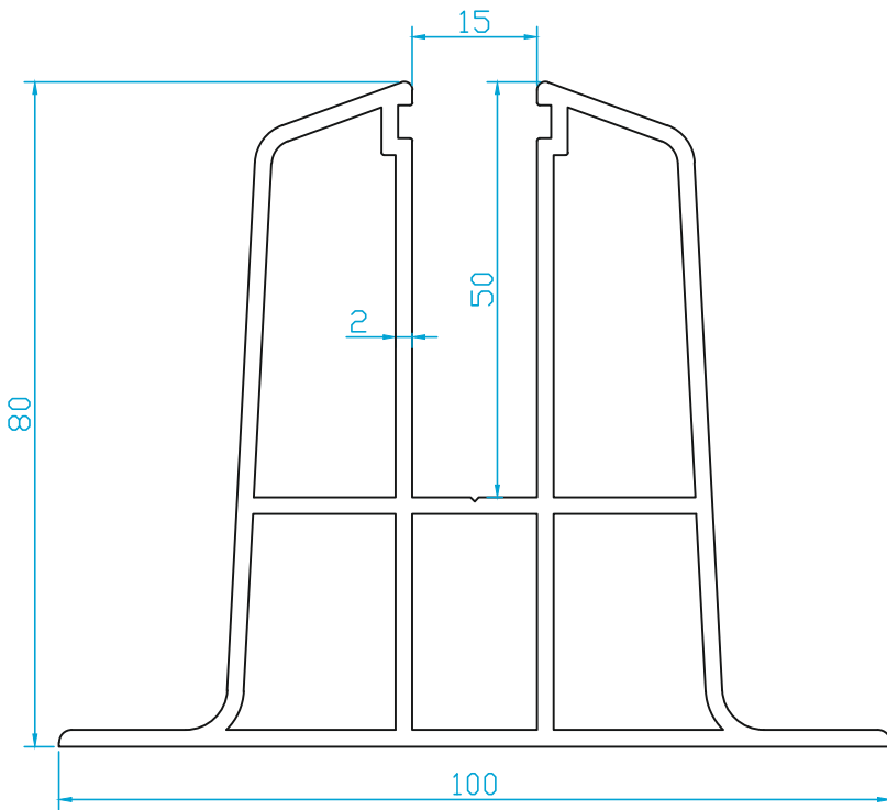
K260 BALKON TABAN PROFİLİ (2.610 Kg/m)
