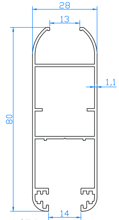
K1674 28x80 SÜRME KANAT TEKCAM (0.800 Kg/m)
