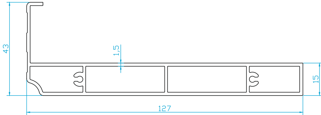
K5811 ALT KASA (GİYOTİN CAMBALKON) 1.485 Kg/m
