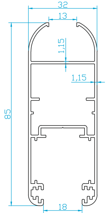
K1671 32x85 SÜRME KANAT (TİJLİ) TEKCAM 0.985 Kg/m
