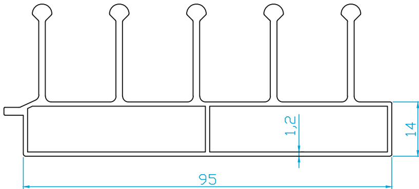
K4469 CAM BALKON SİSTEMİ EŞİKLİ ALT KASA 1.420 Kg/m
