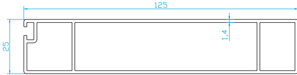
K5473 TENTE ARA KAYIT PROFİLİ (1.320 Kg/m)
