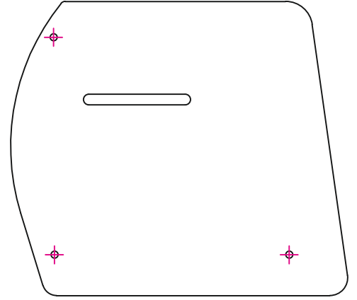
OVAL YAN KAPAK (K5250 İÇİN) (t: 3mm ALÜMİNYUM)
