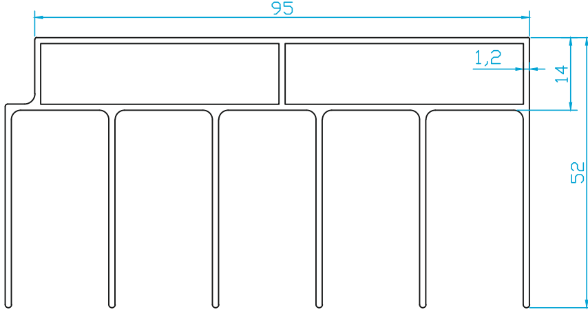
K4457 CAM BALKON SİSTEMİ SÜRME ÜST KASA 1.450 Kg/m
