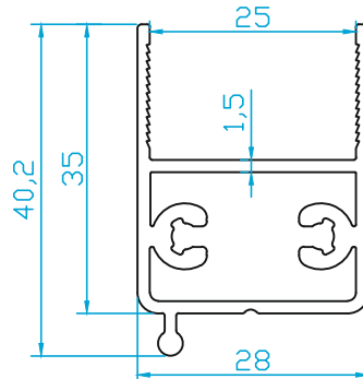
K5814 ÜST BAZA (GİYOTİN CAMBALKON) 0.690 Kg/m
