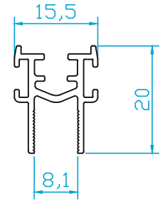
K1852 CAM ÜST FİTİLİ (0.214 Kg/m)
