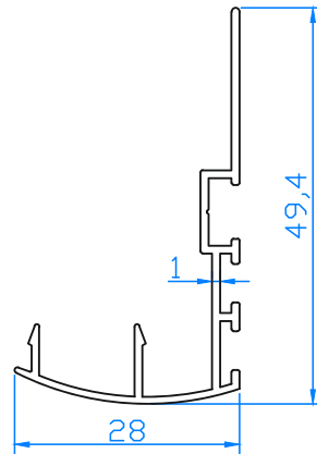
K1675 28x80 SÜRME KENET 0.290 Kg/m
