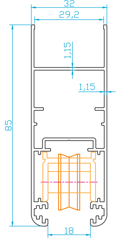
K1670 32x85 SÜRME KANAT (TİJLİ) ÇİFTCAM 0.960 Kg/m
