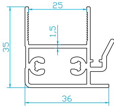
K5813 BAZA (KENET) (GİYOTİN CAMBALKON) 0.800 Kg/m
