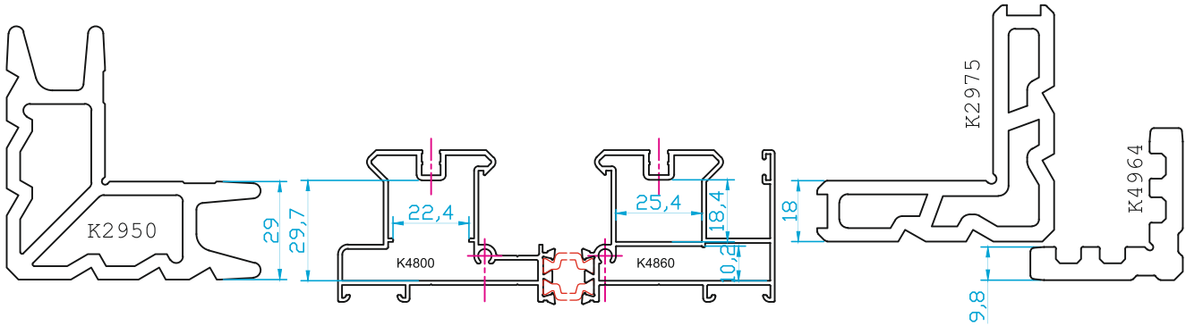
K24680 KALDIR SÜR KASA KÖŞE TAKOZU UYGULAMASI (ÖLÇEK 1/2)
