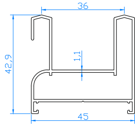
K1679 YALITIMSIZ SÜRME KASA 45 36 mm AKS (0.650 Kg/m)
