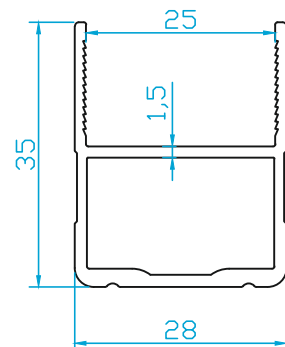
K5816 ALT & YAN BAZA (GİYOTİN CAMBALKON) 0.520 Kg/m
