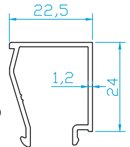
K1654 KALDIR SÜR CAM ÇITASI(22.5) 0.285 Kg/m
