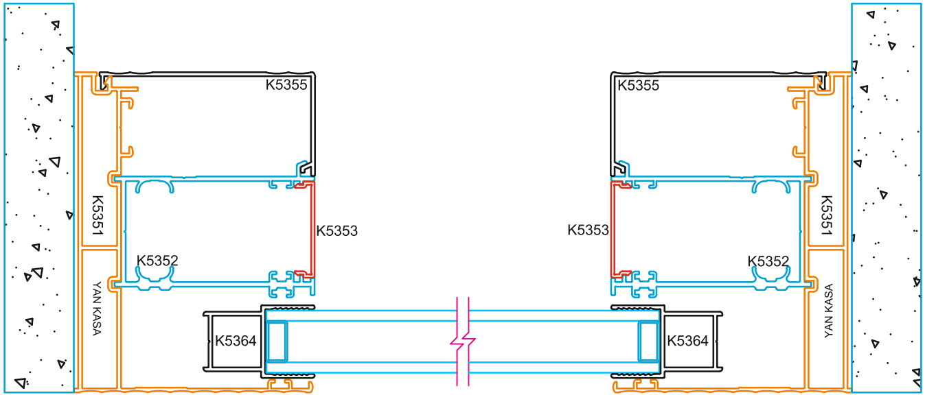
A-A KESİTİ GİYOTİN SİSTEM AÇIK KESİT (YATAY)
