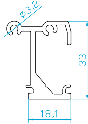
K1996 KAYIT BAĞLANTI PRF. 0.590 Kg/m
