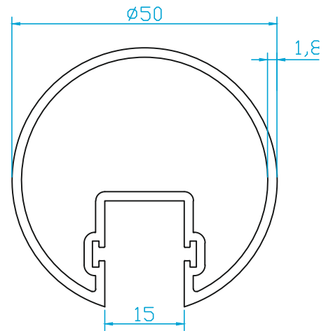
K7750 BALKON ÜST PROFİLİ (0.945 Kg/m)
