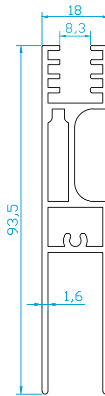
K1620 SÜRME ALT KANAT 1.190 Kg/m
