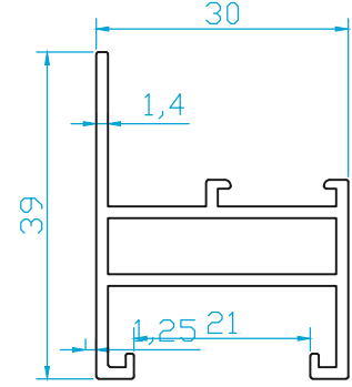
K6735 KANAT (0.495 Kg/m)
