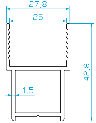
K5364 ASKİ PROFİLİ (JALUZİ CAM) (0.520 Kg/m)
