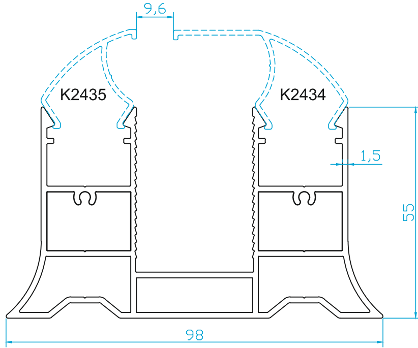
K2433 BALKON TABAN PROFİLİ (1.875 Kg/m)
