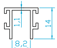
K4497 CAM TUTUCU 8 mm 0.157 Kg/m
