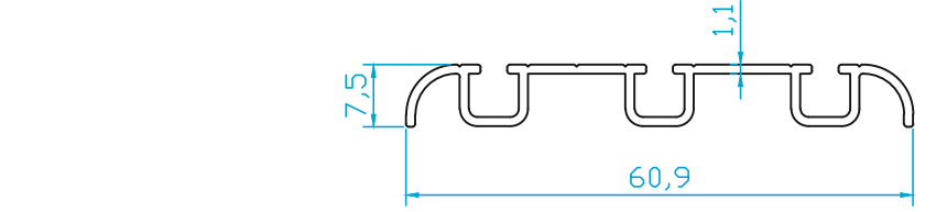
K4462 EŞİKSİZ ALT KASA (3LÜ) 0.340 Kg/m
