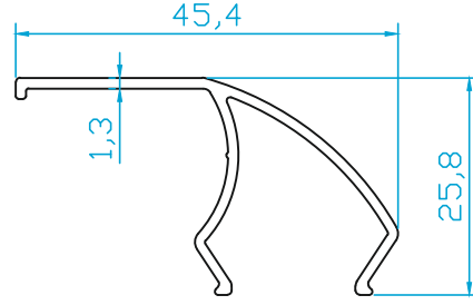
K2434 BALKON ÇİTA 0.300 Kg/m
