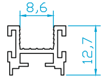
K4496 CAM KARŞILIK 8 mm 0.165 Kg/m
