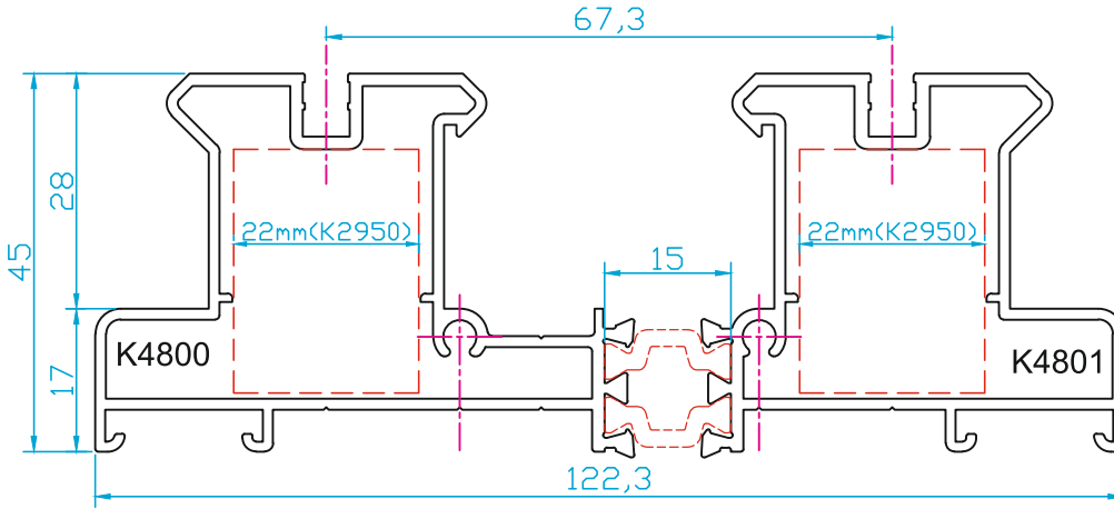
K24800 KALDIR SÜR KASA (TAKIM SiP.NR: K24800) 2.050 Kg/m (ISI BARIYERLİ)
