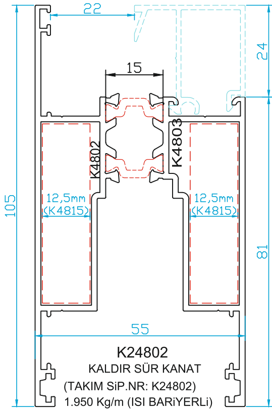
K4835 PERVAZ 0.275 Kg/m
