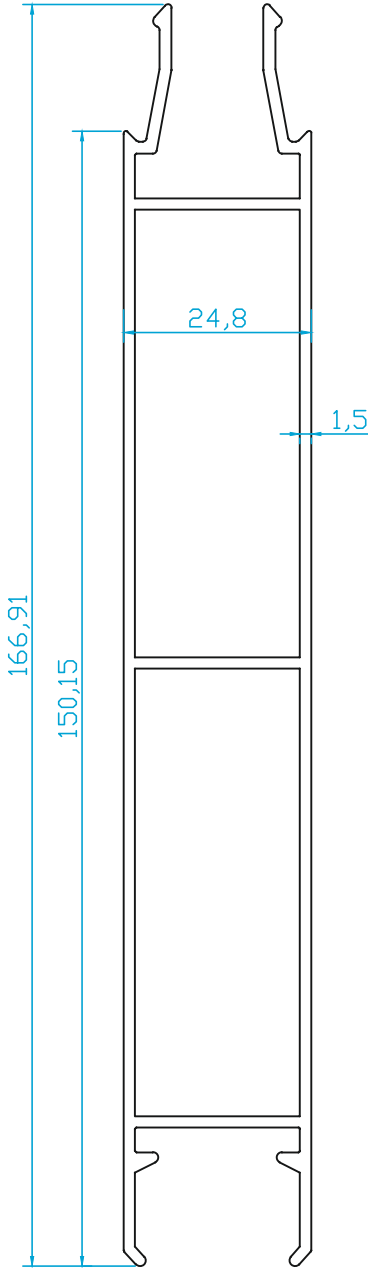
K1340 Aluplanke 1.710 Kg/m
