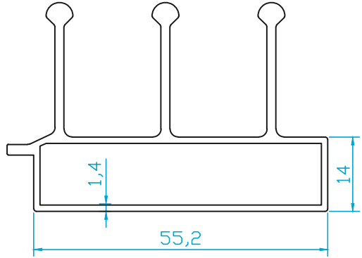
K4461 EŞİKLİ ALT KASA (3LÜ) 0.900 Kg/m
