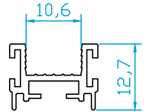
K4747 CAM KARŞILIK 10 mm 0.170 Kg/m
